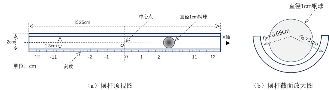
图 3 摆杆结构示意图
