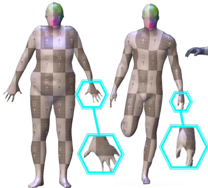
Anisotropic
