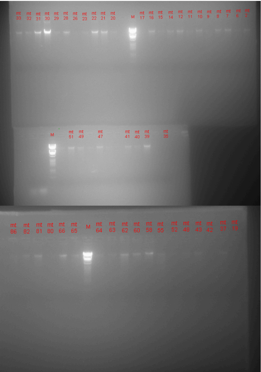
普通琼脂糖凝胶电泳：lambda双切上样5μl。样品上样量为 5μl。
