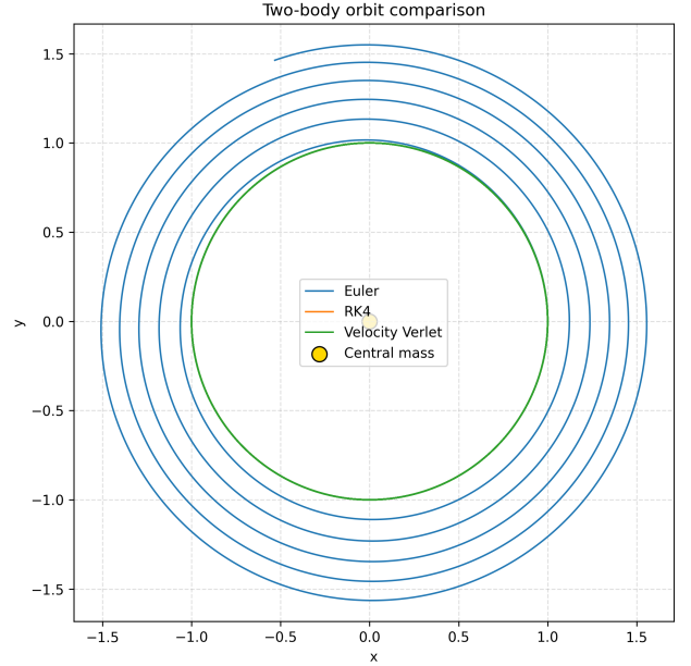
图 1 不同积分方法得到的两体轨道比较。
