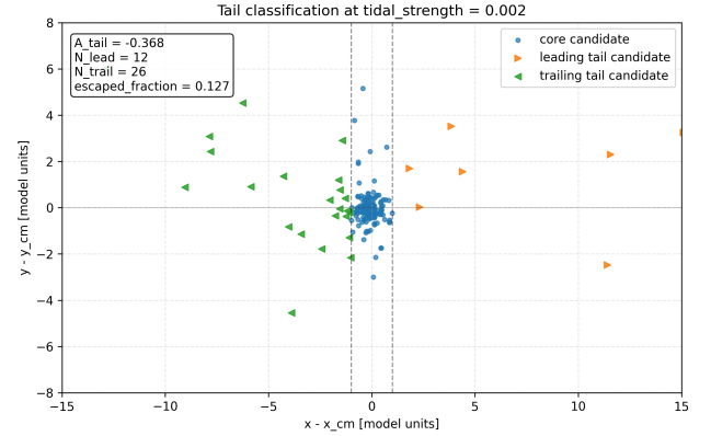
图6 最终快照中核心与潮汐尾候选粒子的简单分类。
