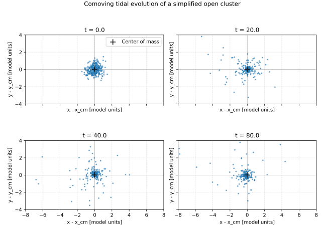
图5 温和潮汐场下星团在质心系中的长期演化。
