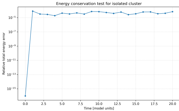
图4 孤立星团中 Velocity Verlet 方法的能量守恒测试。
