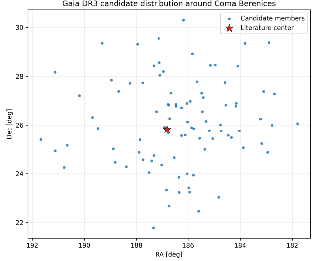
图 9 Gaia DR3 中 Coma Berenices 候选成员的天球分布。
