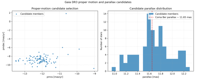
图 10 Gaia DR3 候选成员的自行分布和视差分布。
