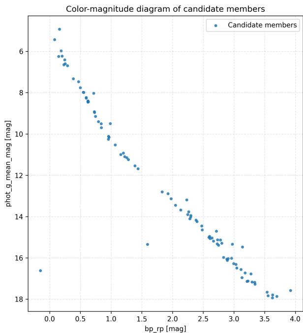
图 11 Gaia DR3 候选成员的颜色星等图。
