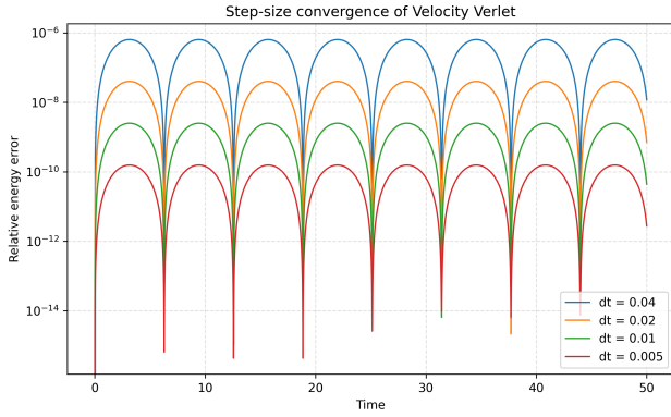
图3 Velocity Verlet 方法的步长收敛测试。
