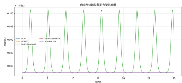
图 18 欧拉角的数值解, 隐式中点辛积分能量误差呈现周期性且非常大, 我们在尝试不同总角动量和不同时间长短之后效果一致。
