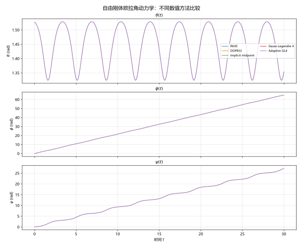
图 17 欧拉角的数值解, 与相图中的转动状态一致。
