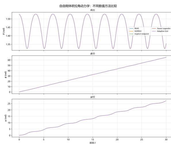
图 17 欧拉角的数值解, 与相图中的转动状态一致。
