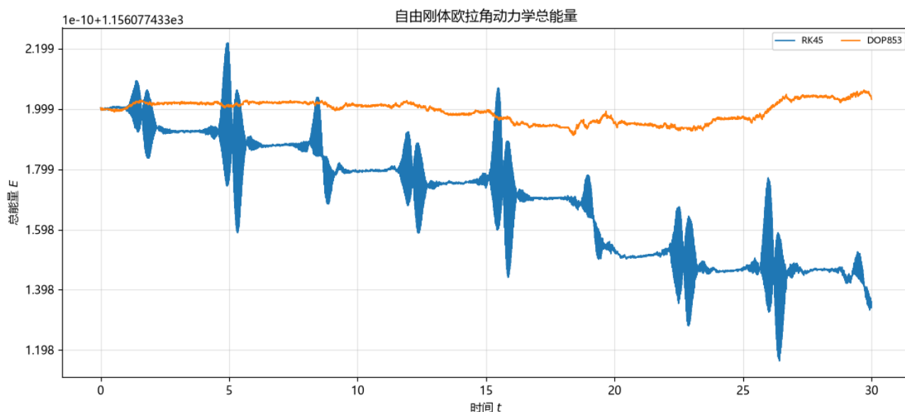
图 16 进一步去除所有辛方法的曲线, RK45 特征与前面的图差不多, 但是量级远小于辛方法, 同时表现最为优秀的是 DOP853, 其能量变化有非单调的特征存在, 加之其误差本就很小, 使其能量变化相当少.
