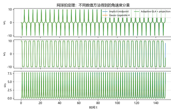
图 14 长时间后的情况, 没有显著区别, 并且能量近乎不变, 能量图像仅为一条直线, 在有意义的范围内几乎无波动。
