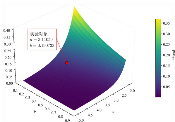
图 7 \varepsilon_0 的数值解可视化 3D 图, 可以看出, 当 a 和 b 越小 ( I_1, I_2, I_3 越接近), \varepsilon_0 越大, 本文章的实验对象的相关数据已在图中标出。
