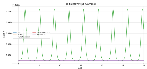
图 18 欧拉角的数值解, 隐式中点辛积分能量误差呈现周期性且非常大, 我们在尝试不同总角动量和不同时间长短之后效果一致。
