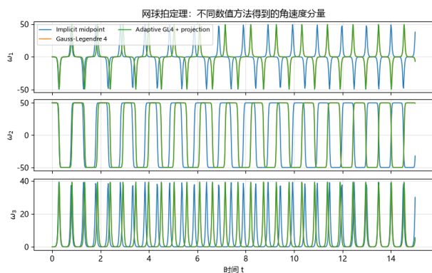
图 15 增大初始值的情况, 在一段时间后算法预测的角速度结果出现劈裂 (橙线和绿线是重合的), 能量仍然很好地被保持了。
