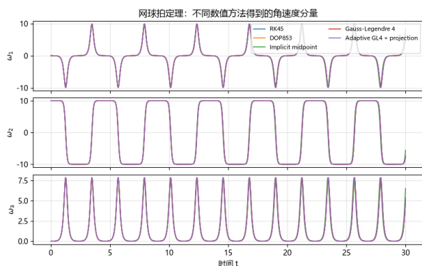
图 13 多种算法绘制出的系统演化图像, 良好的重合了。
