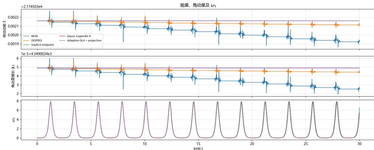
图 12 能量图像, 在能量和角动量图中我们把角动量中的 \omega_3 放到了里面, 高阶自适应步长算法在剧烈变化 (指数级增长和衰减) 的时候呈现的能量波动以及波动后的能量的变化十分显著且对应关系明确。
