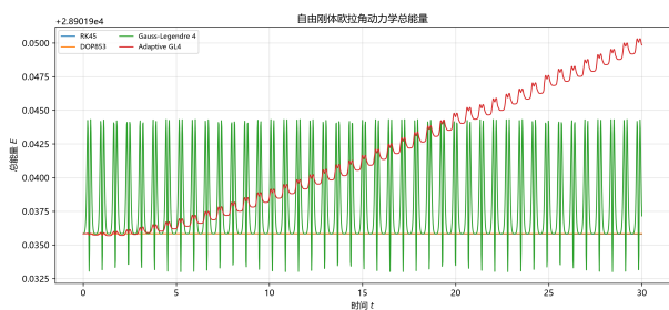
图 20 提高初值大小, 我们发现此处 GL4 的误差对于初值的大小十分敏感, 这可能是由于其精度阶数很低导致快速变化对其的冲击远大于其他算法, 而 Adaptive GL4 由于有自适应步长, 就很好地减少了此冲击的效果.
