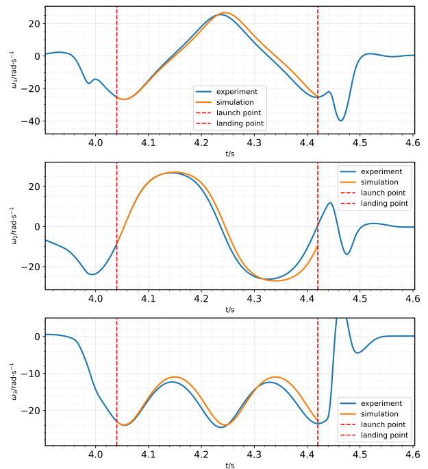
图 4 数值模拟以及实验数据对比-中间轴.
