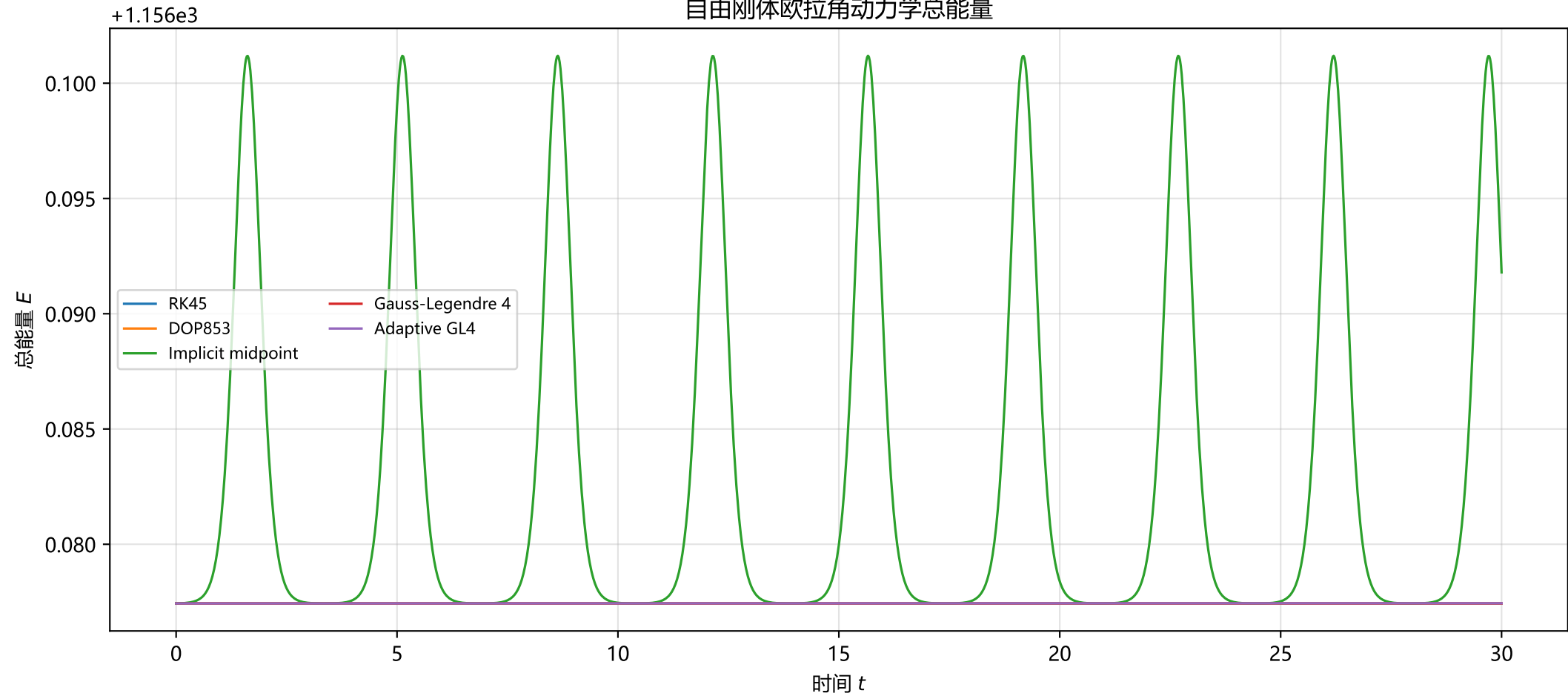
自由刚体欧拉角动力学总能量
