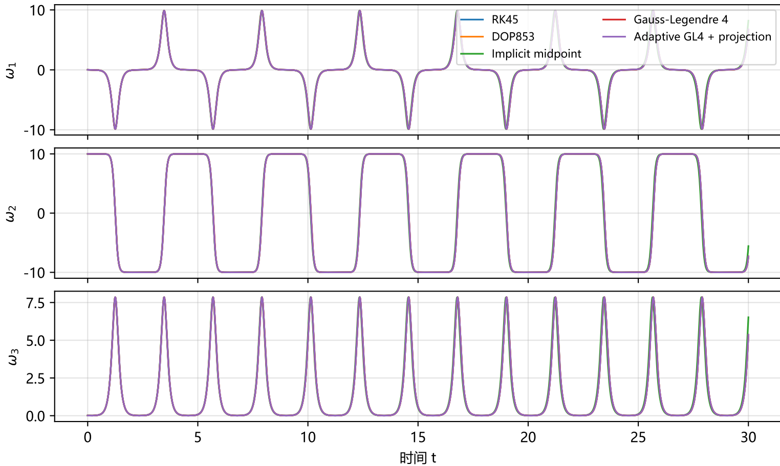
网球拍定理：不同数值方法得到的角速度分量
