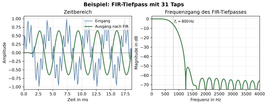
Abbildung 2.3: Beispiel eines FIR-Tiefpasses mit 31 Filterkoeffizienten und einer Grenzfrequenz von f_c = 800 Hz. Der Filter arbeitet ohne Rückkopplung und dämpft hohe Frequenzanteile. Eigene Darstellung nach (Smith, 2007).
