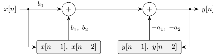
(a) Direktform I: zwei Verzögerungsketten, vier gespeicherte Werte
