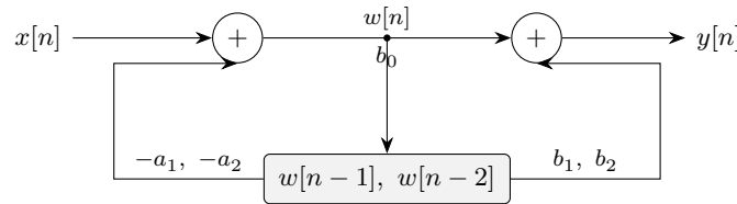
(b) Direktform II: eine Verzögerungskette, zwei gespeicherte Werte
