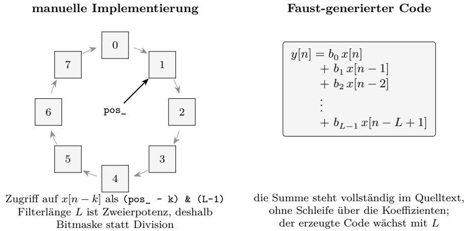
Abbildung 5.3: Zwei Wege zur selben Faltung. Die manuelle Implementierung hält die vergangenen Eingangswerte in einem Ringpuffer und läuft in einer Schleife über die Koeffizienten. Der Faust-Compiler schreibt dieselbe Summe vollständig aus.
