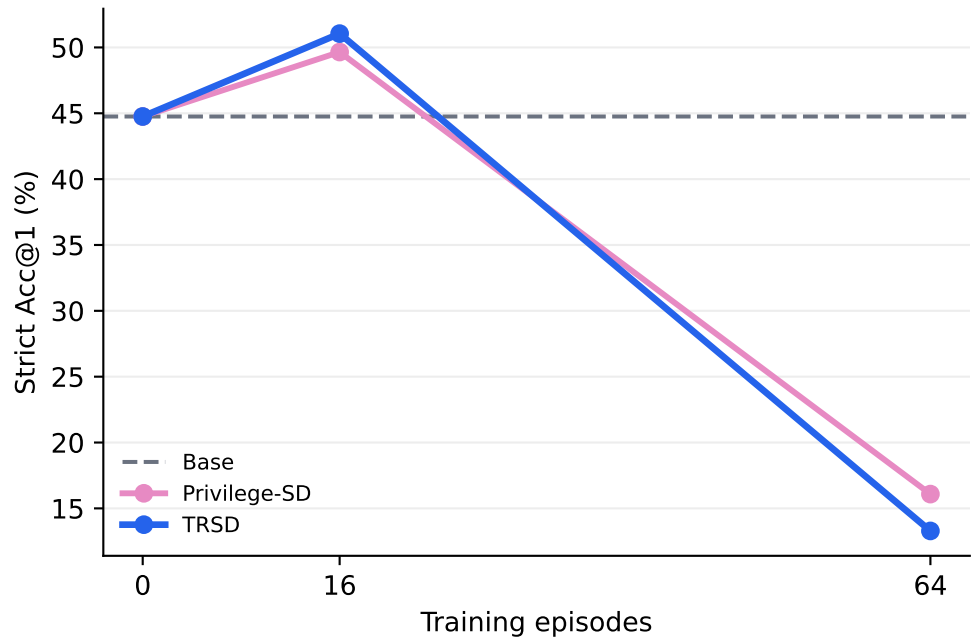
Qwen3-1.7B
