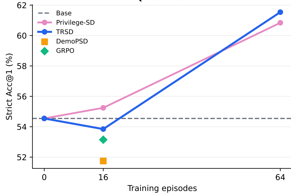
Qwen3-8B
