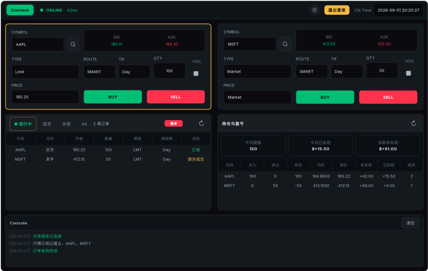
Client 主交易界面：双交易栏、报价、订单、持仓与控制台。
