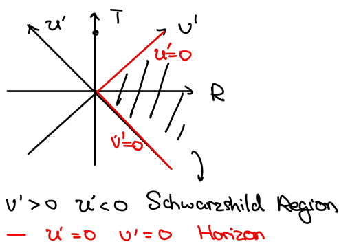
图 12: Kruskal 坐标系下的时空结构图
