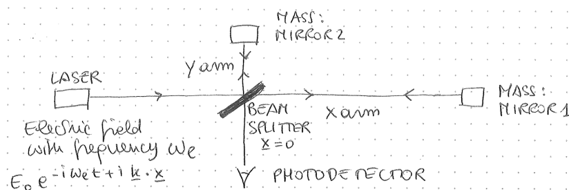
图 2: Interferometer 的结构示意图
