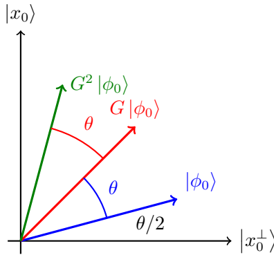
Figure 3: Grover 迭代的几何图像 (取 \theta/2 = 15^\circ 示意): 状态在 \text{span}\{|x_0\rangle, |x_0^\perp\rangle\} 内每次旋转角度 \theta ; 初态 |\phi_0\rangle 与 |x_0^\perp\rangle 的夹角为 \theta/2 , 迭代 k 次后夹角为 (2k+1)\theta/2 , 逐步趋向标记态 |x_0\rangle .
