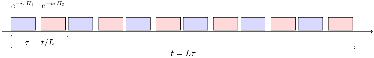
Figure 4: 一阶 Trotter 乘积公式: 时间区间 [0, t] 划分为 L 步, 每步交替演化 e^{-i\tau H_1} 与 e^{-i\tau H_2} ; 单步误差 O(\tau^2) , 经 L 步累积为 O(L\tau^2) = O(t^2/L) .
