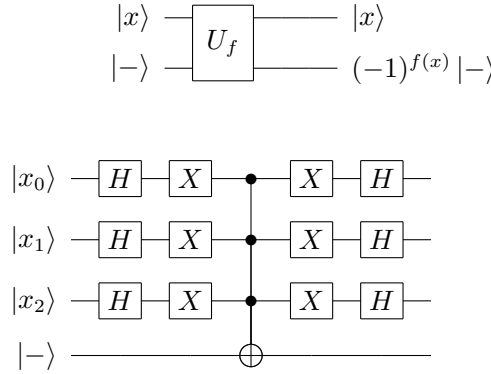
Figure 2: Grover 迭代电路. 上图: 相位反冲 ——辅助比特取 |-\rangle 时, 比特 oracle U_f |x\rangle |y\rangle = |x\rangle |y \oplus f(x)\rangle 等价于相位 oracle U_f |x\rangle = (-1)^{f(x)} |x\rangle (标记态被附加 -1 相位). 下图: 扩散算子 R_0 = 2|\phi_0\rangle\langle\phi_0| - I = H^{\otimes 3}(2|0^3\rangle\langle 0^3| - I)H^{\otimes 3} 的显式实现 ( n = 3 示意): X^{\otimes 3} 把 2|0^3\rangle\langle 0^3| - I 化为对 |1^3\rangle 的相位翻转, 再以 |-\rangle 辅助比特为目标的 C^3NOT 实现之 (三个控制点经竖线指向同一目标). 每次迭代后辅助比特回到 |-\rangle , 可复用.
