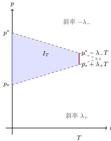
Figure 1: 恢复定理的几何: 误差初值为零的区间 (p_*, p^*) 在 p -方向以速度至多 \lambda_+ (向右) 与 \lambda_- (向左) 收缩, 到时刻 T 干净区间收缩为 I_T = (p_* + \lambda_+ T, p^* - \lambda_- T) (红色竖线段), 其上 w(T, p) = e^{-p} u(T) . 热方程型 ( H_1 \leq 0 ) 时 \lambda_+ = 0 , 左边界不动, 仅右边界以 \lambda_- 收缩; 全耗散 ( \lambda_{\pm} = 0 ) 时 I_T = (p_*, p^*) 永不收缩. 图取 \lambda_+ = \lambda_- = 0.3 .
