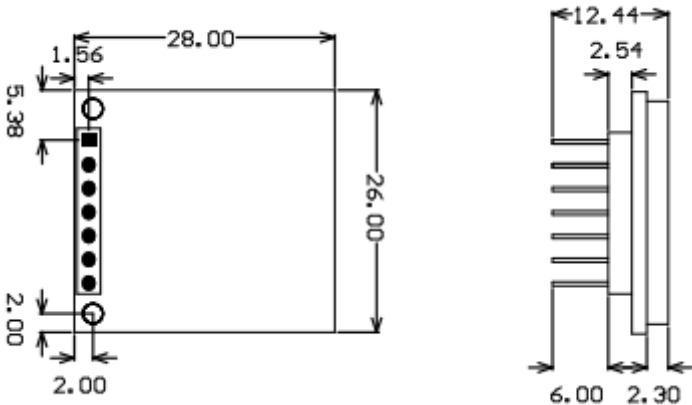
单位 mm 误差+/-0.2mm
