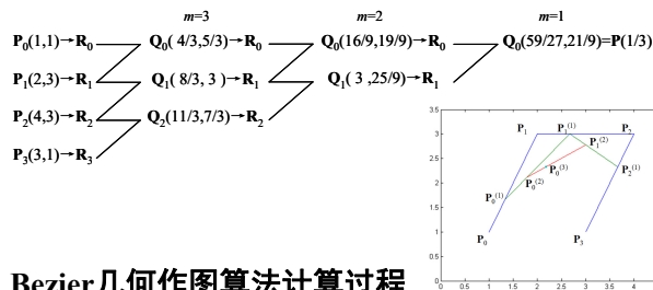
Bezier几何作图算法计算过程
