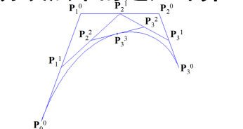
分裂法的示意图
