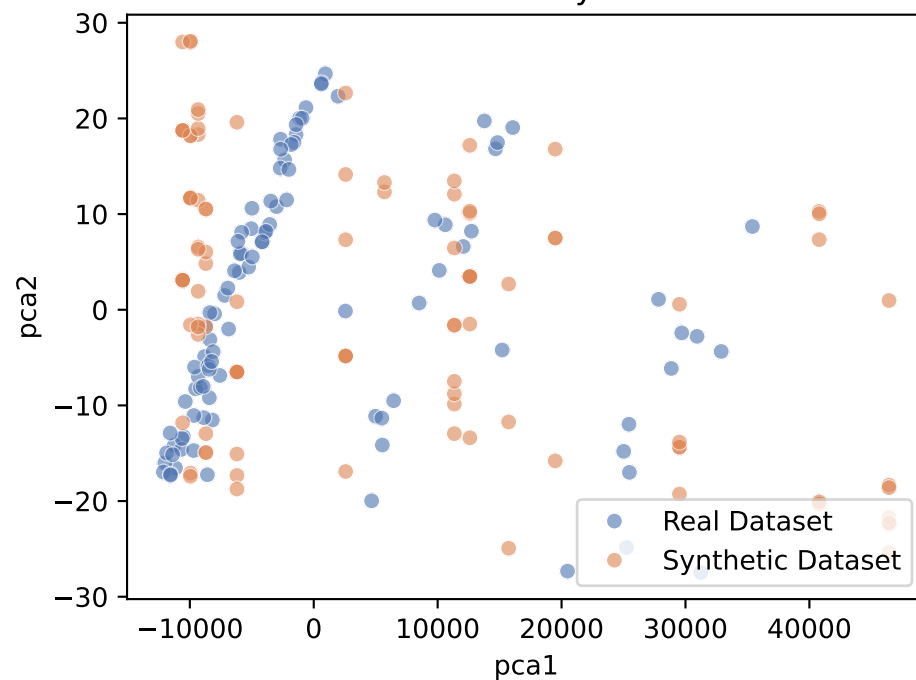
FedPrivSyn
