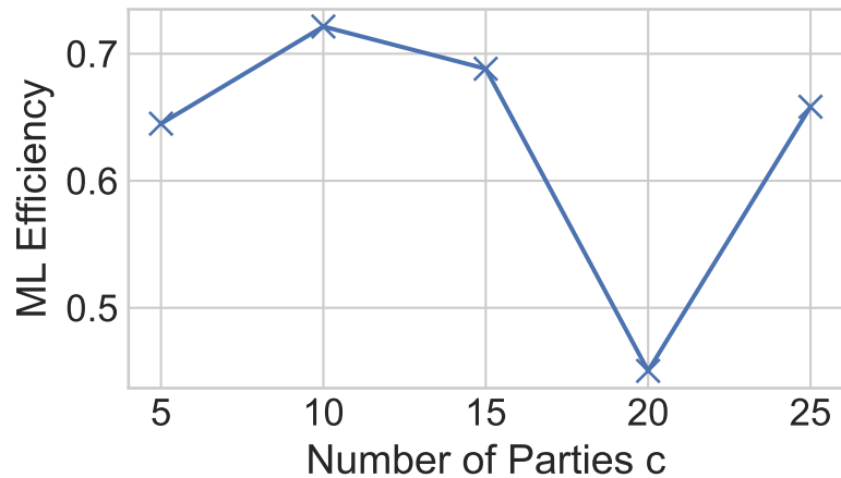
AdaFedPrivSyn
