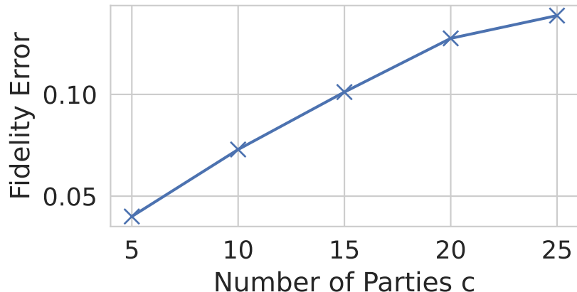
AdaFedPrivSyn
