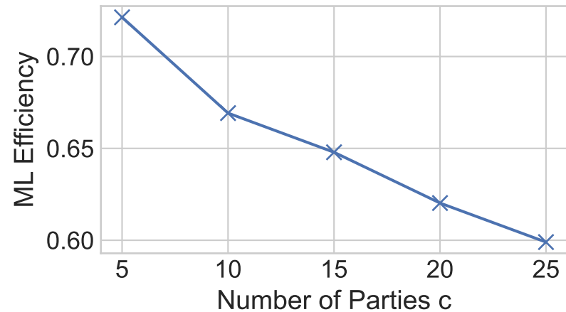
FedPrivSyn
