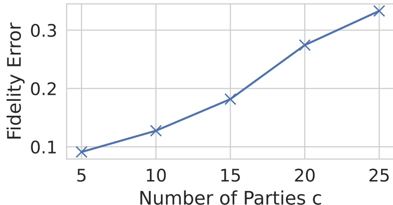
FedPrivSyn
