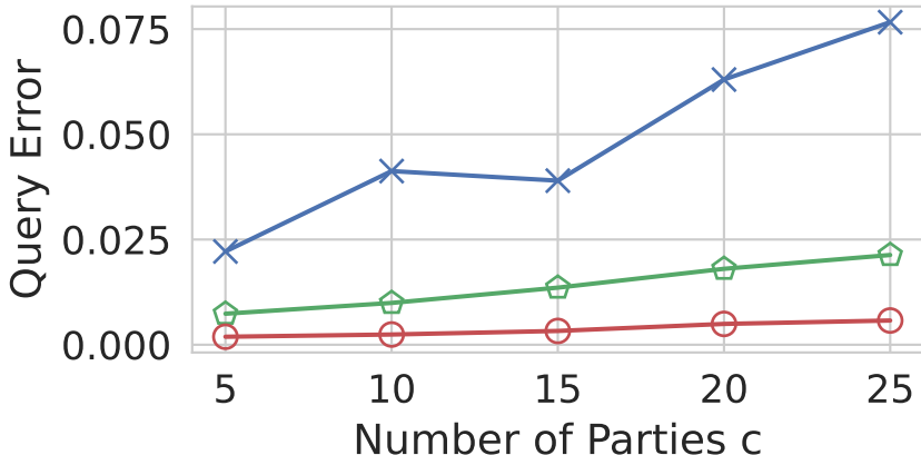
FedPrivSyn
