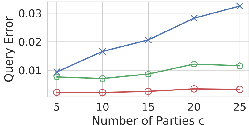
AdaFedPrivSyn
