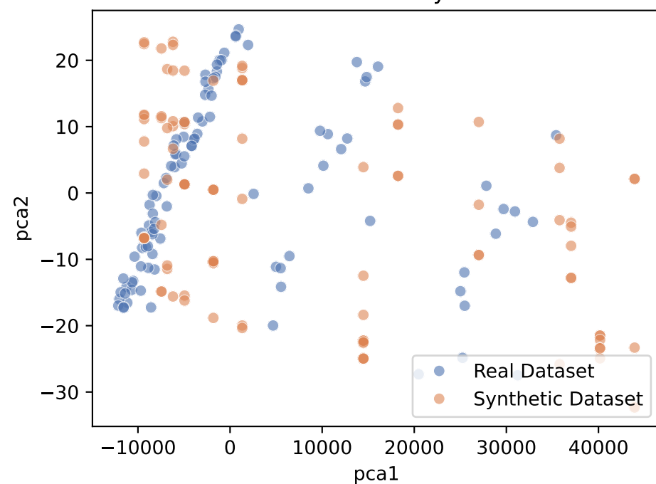
AdaFedPrivSyn
