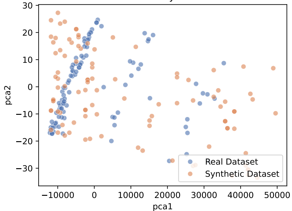
PrivSyn
