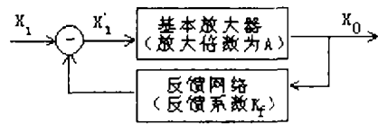
图 1 系统示意
