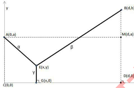
图 3 有共用管线时的设计图
