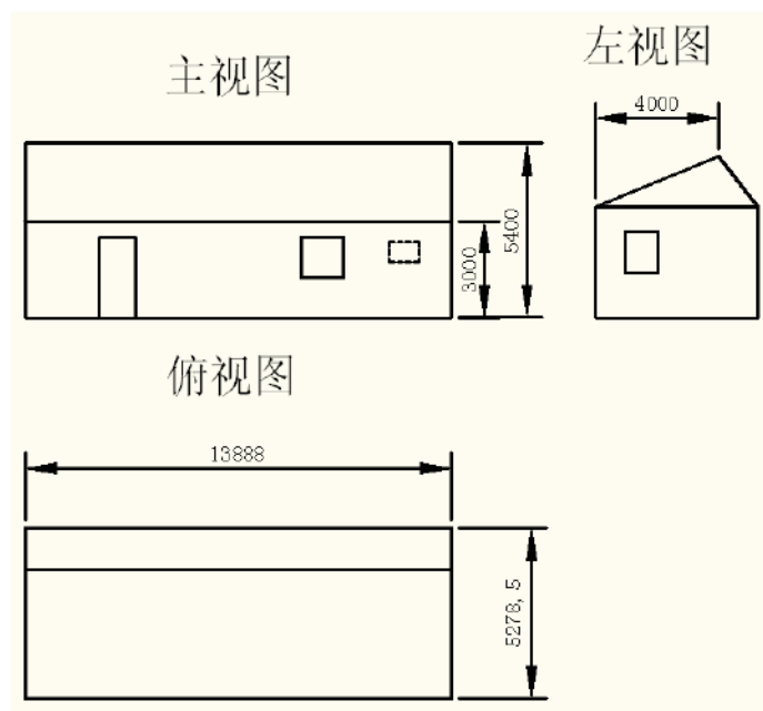
图 15 小屋设计图
