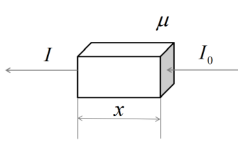
图 2: Lambert-beer吸收定律示意图
