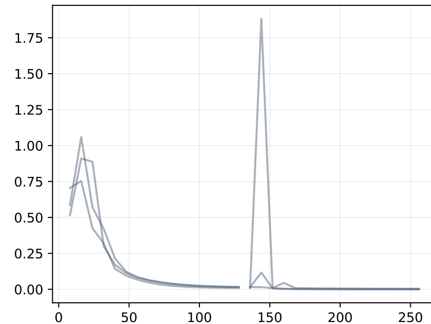
SFT token CE
