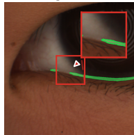
DeepLabV3
