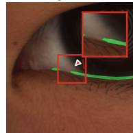
DeepLabV3
