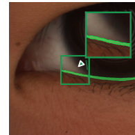
GAL-SAM (Ours)
