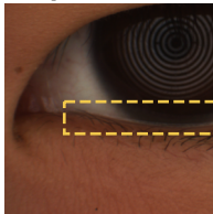
Input (YOLO)
