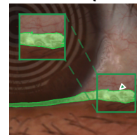
GAL-SAM (Ours)
