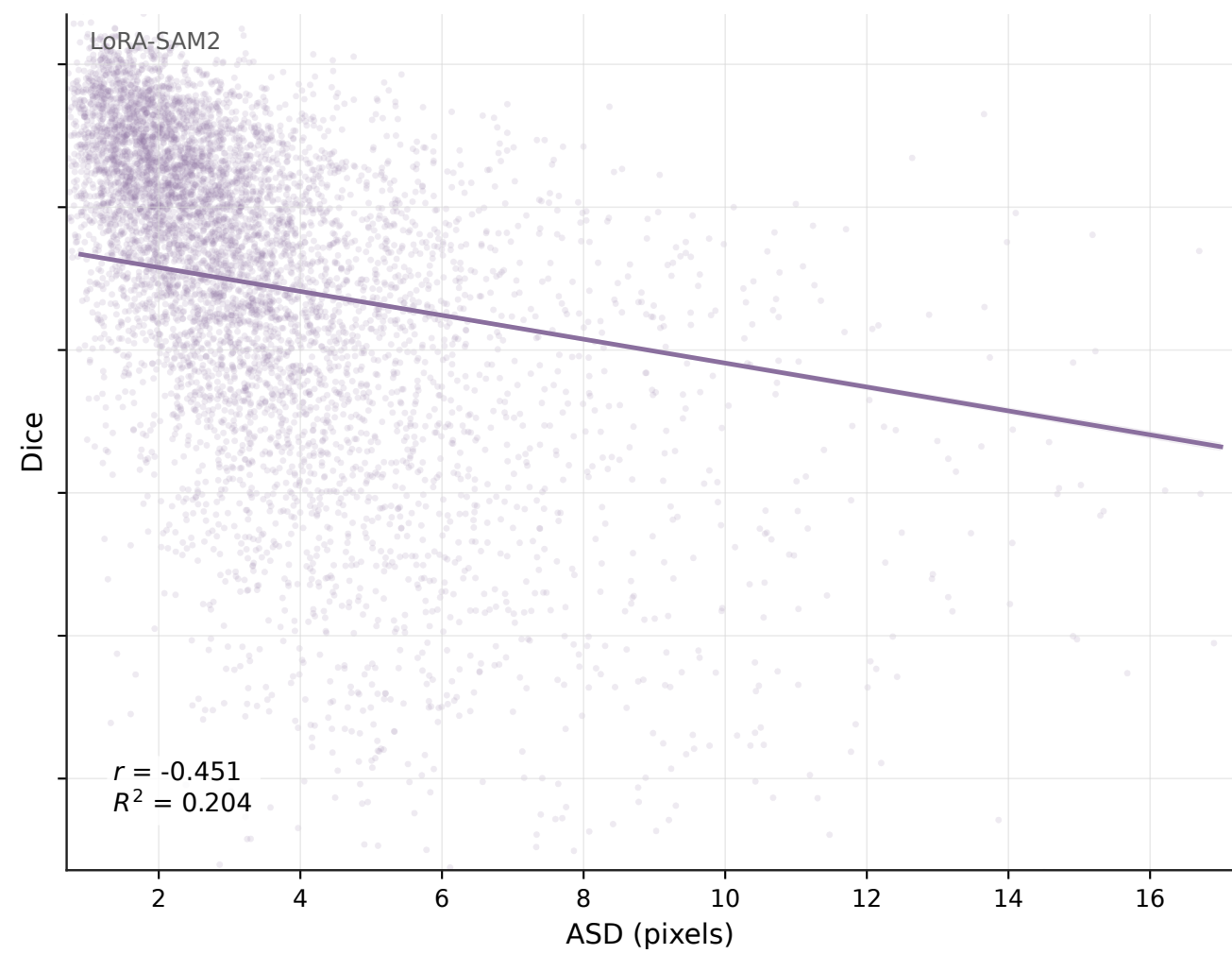
LoRA-SAM2
