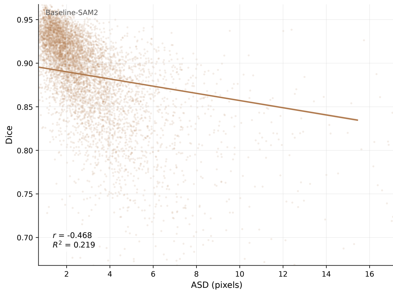
Baseline-SAM2
