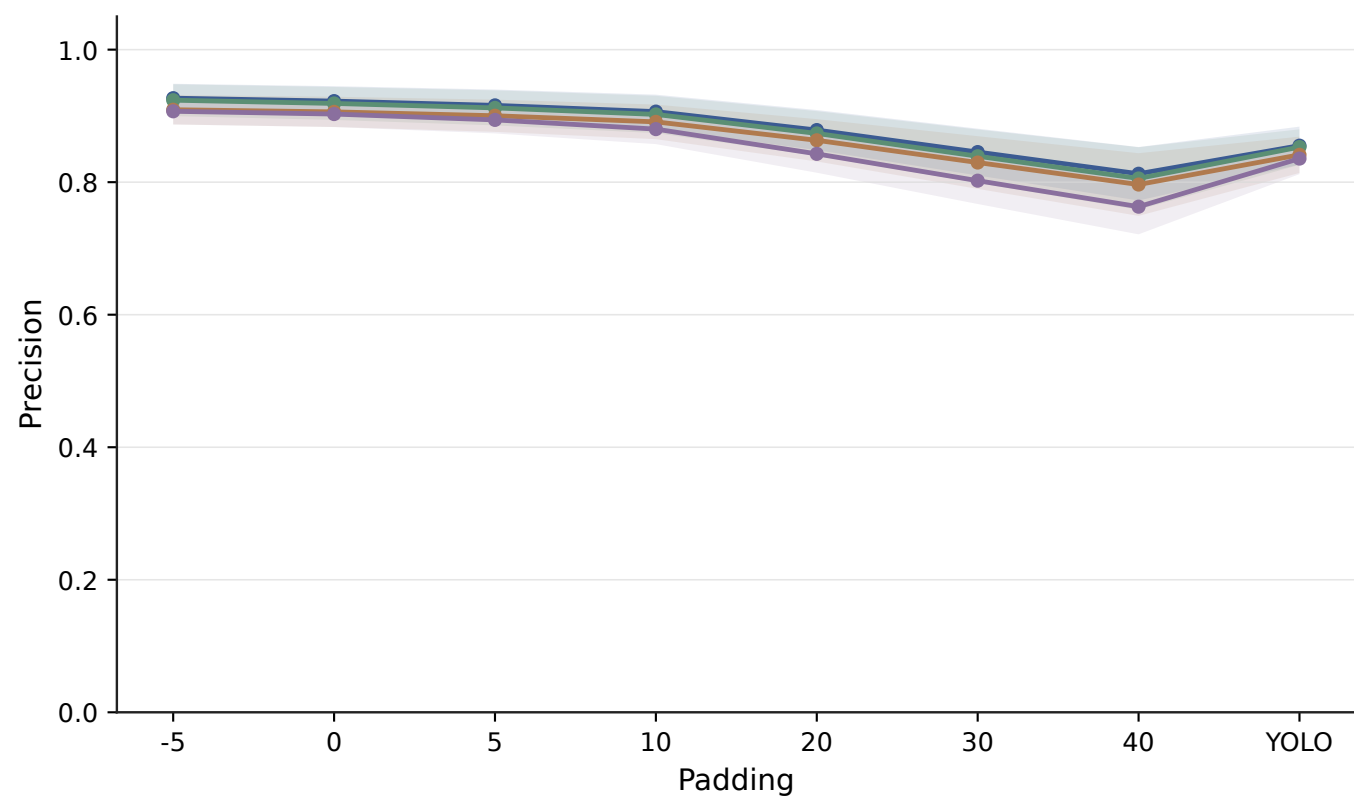
Precision
