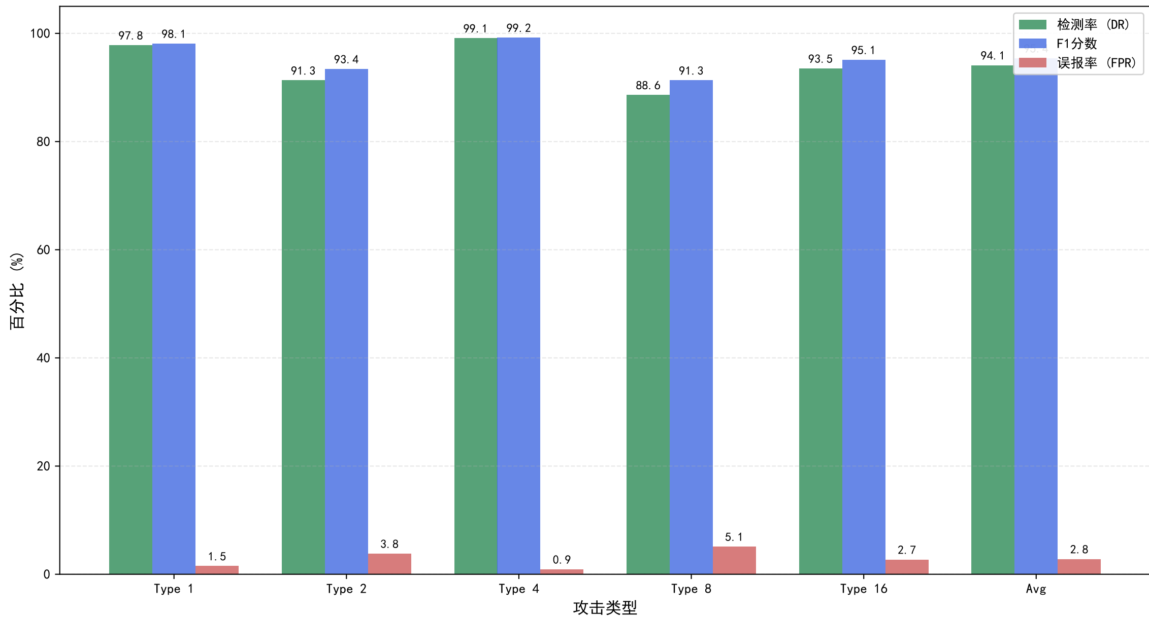
SAFL-VR对不同攻击类型的检测性能
