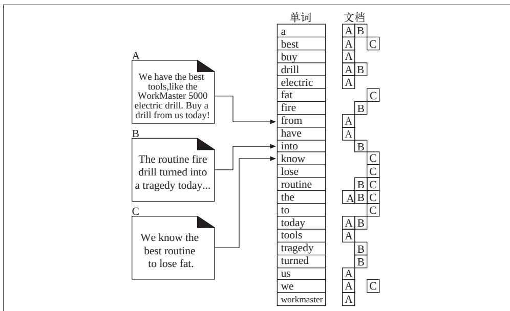
图 9-8 三份文档和一个全文索引
