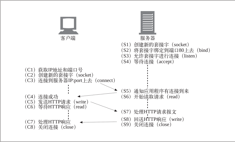
图 4-6 TCP 客户端和服务是如何通过 TCP 套接字接口进行通信的
