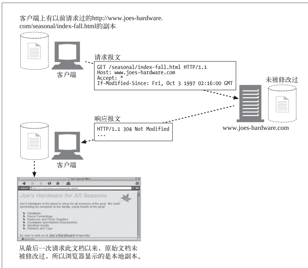
图 3-15 重定向为使用本地副本的请求
