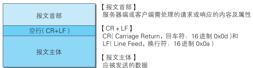
图：HTTP 报文的结构
