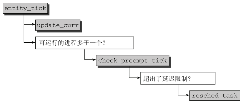
图2-22 entity_tick的代码流程图
