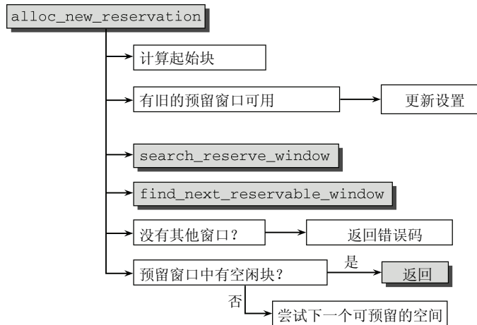
图9-17 alloc_new_reservation 的代码流程图
