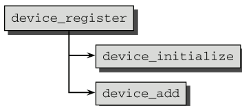
图6-22 device_register 的代码流程图
