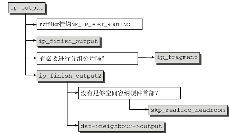
图12-19 ip_output的代码流程图
