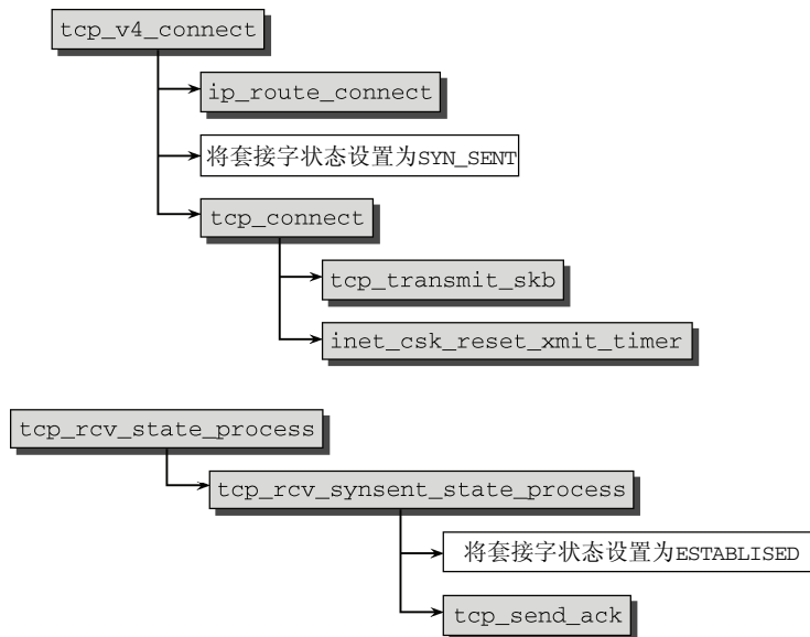
图12-29 主动的连接建立的代码流程图
