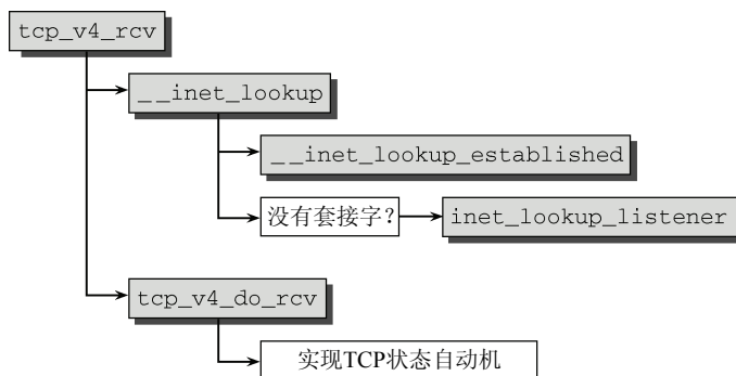
图12-27 tcp_v4_rcv的代码流程图
