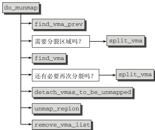
图4-13 do_munmap 的代码流程图
