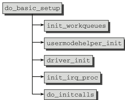
图D-4 do_basic_setup 的代码流程图
