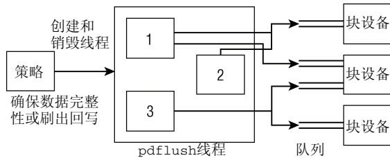
图17-2 pdflush机制概述
