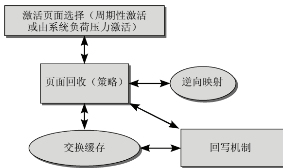
图18-4 交换缓存和页交换子系统的其他组件的交互
