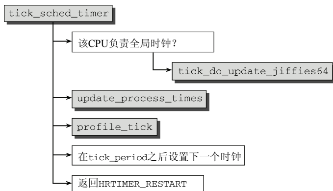
图15-17 tick_sched_timer的代码流程图
