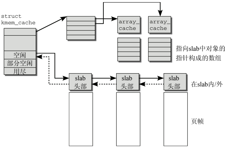
图3-45 slab缓存的精细结构
