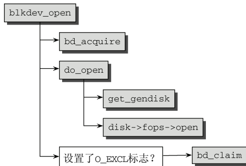
图6-13 blkdev_open的代码流程图
