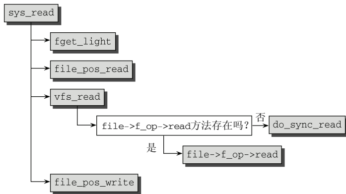
图8-12 sys_read的代码流程图
