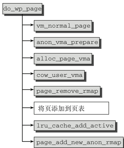
图4-20 do_wp_page的代码流程图
