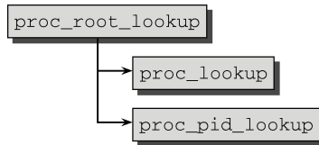
图10-3 proc_root_lookup 的代码流程图
