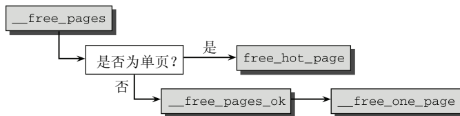
图3-35 __free_pages 的代码流程图
