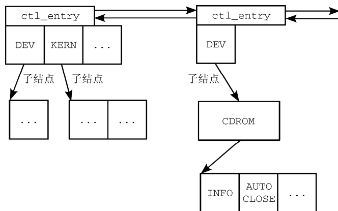
图10-7 ctl_table_header和ctl_table之间的关系
