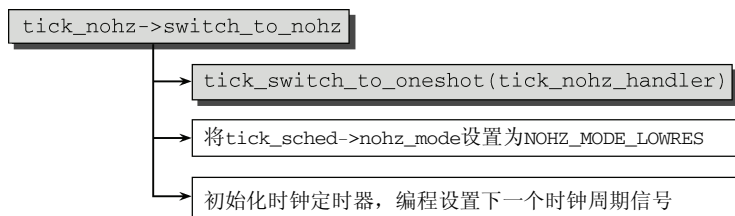
图15-19 tick_nohz_switch_to_nohz 的代码流程图
