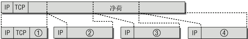
图12-20 IP分组分片
