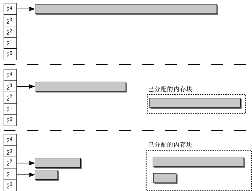
图1-8 伙伴系统
