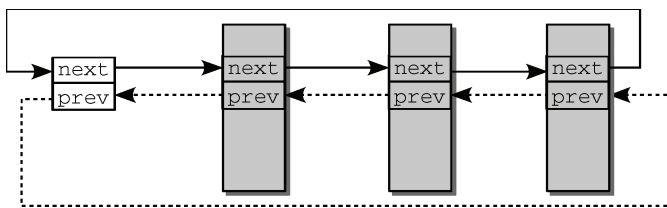
图1-11 标准双链表
