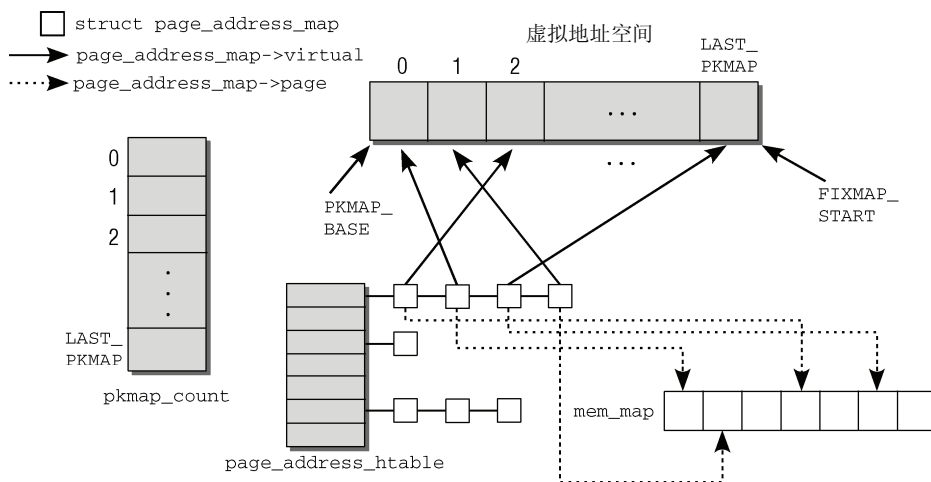
图3-41 用于管理持久映射的数据结构
