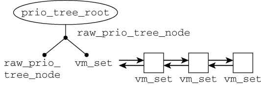
图4-9 管理共享的相同映射所涉及各个数据结构的关联
