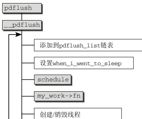
图17-3 pdflush的代码流程图
