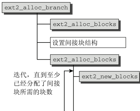
图9-12 ext2_alloc_branch的代码流程图
