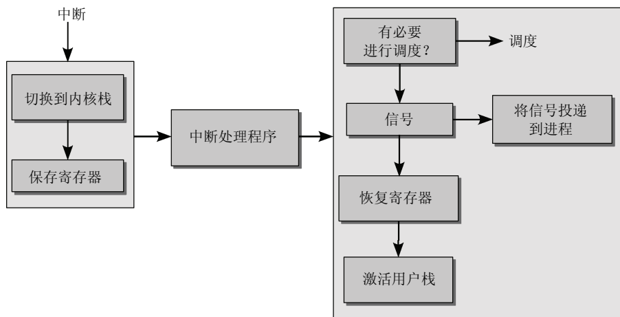
图14-2 中断的处理
