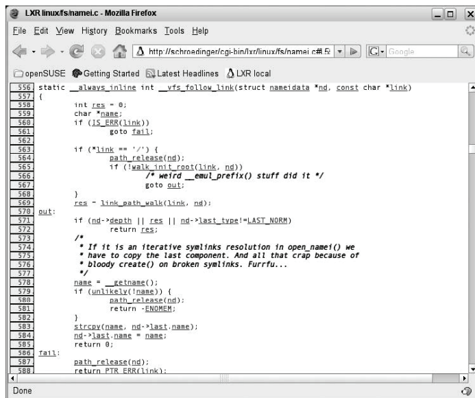
图B-4 通过LXR生成的超文本来查看Linux源代码
