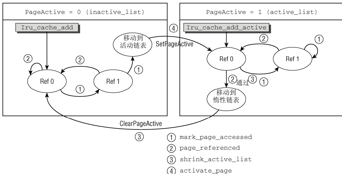
图18-13 就PG_active和PG_referenced标志位而言，内存页可能状态迁移的概述，以及页如何相应地放置到活动链表或惰性链表上
