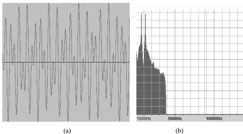
图 15-9 按键“1”对应的音频在时域和频域的形态
