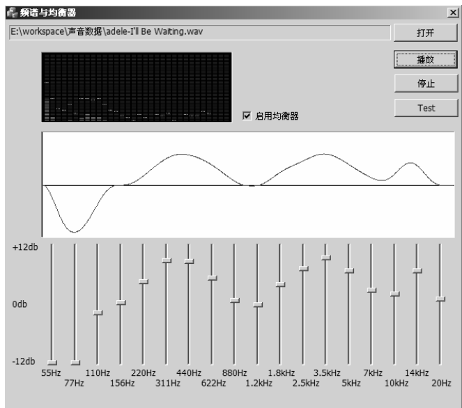
图 15-10 一个仿 Foobar 的 18 段均衡器的例子
