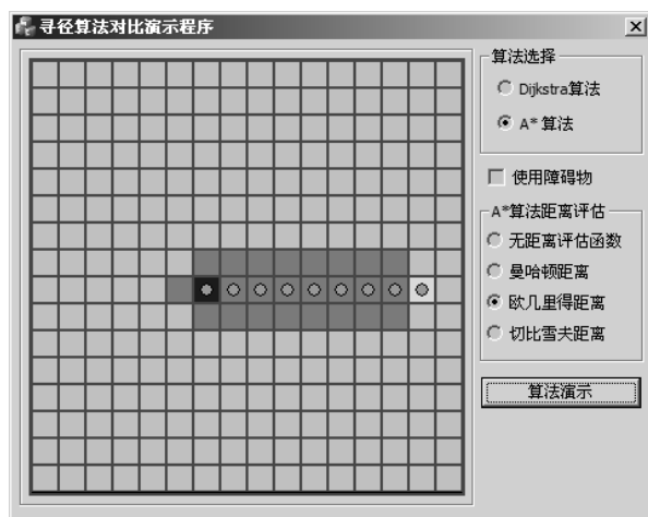
图 21-5 在没有障碍物的情况下，欧几里得距离评估函数的效果
