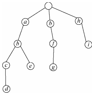
图 2-3 字典树示意图
