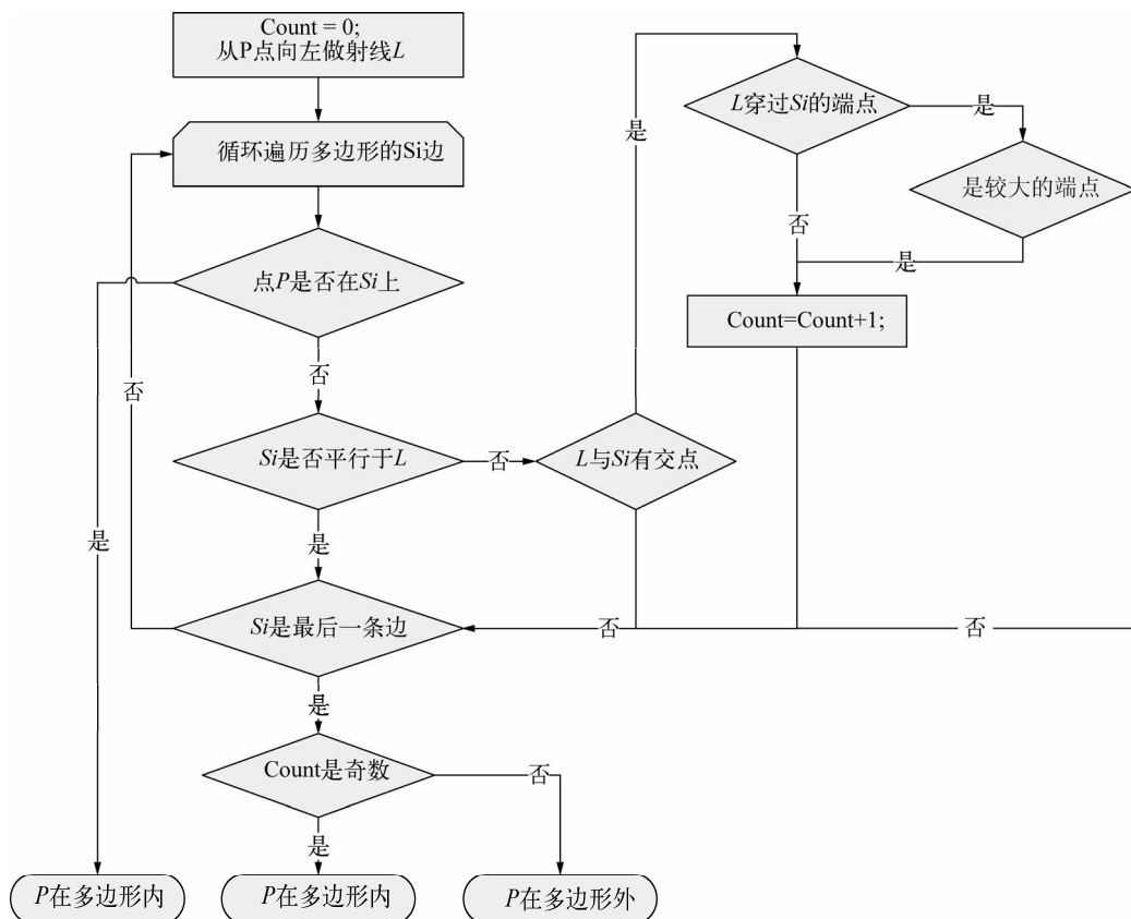
图 14-5 判断点是否在多边形内的扫描线算法流程
