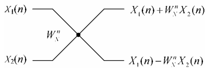
图 15-3 蝶形运算关系图
