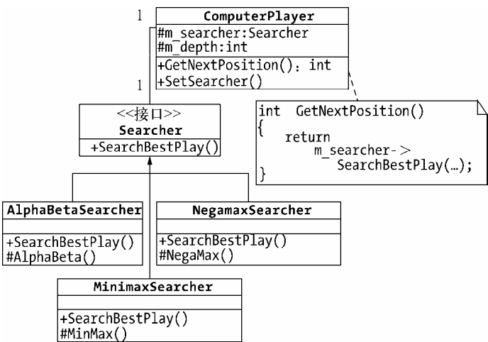
图 B-2 计算机玩家与搜索算法关系图
