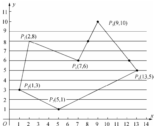
图 14-20 多边形与扫描线示意图
