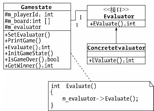
图 B-3 GameState 与评估算子 Evaluator 关系图
