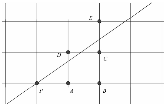
图 14-8 直线两步算法示意图
