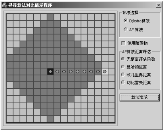
图 21-1 Dijkstra 算法搜索效率图示（无障碍物的情况）
