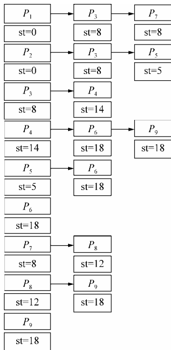
图 9-4 图的邻接表表达形式
