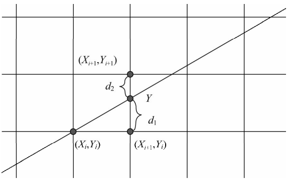
图 14-7 直线 Bresenham 算法示意图
