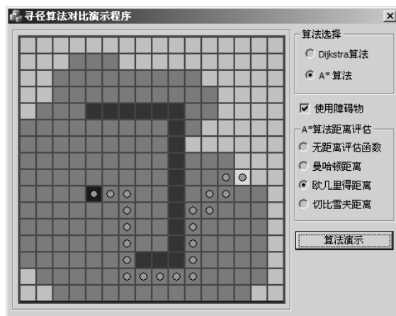
图 21-7 使用欧氏几何平面距离的 A*算法效果
