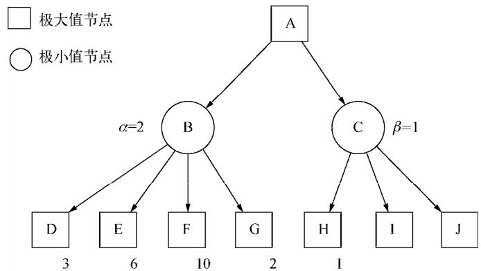
图 23-2 “ \alpha 剪枝” 过程示意图
