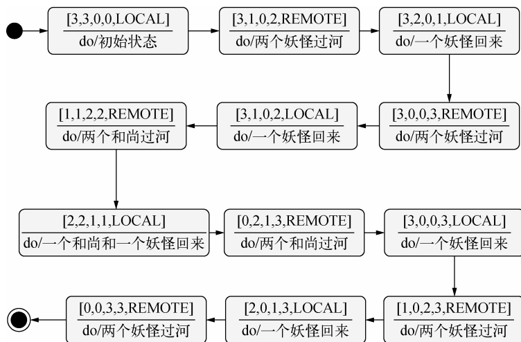
图 6-2 一个过河结果的状态转换过程
