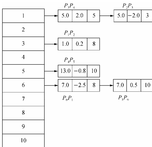
图 14-22 各扫描边的新边表
