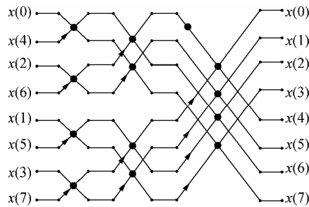
图 15-4 8 点 FFT 蝶形运算位置关系图
