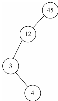
图 2-2 退化为链表的二叉排序树
