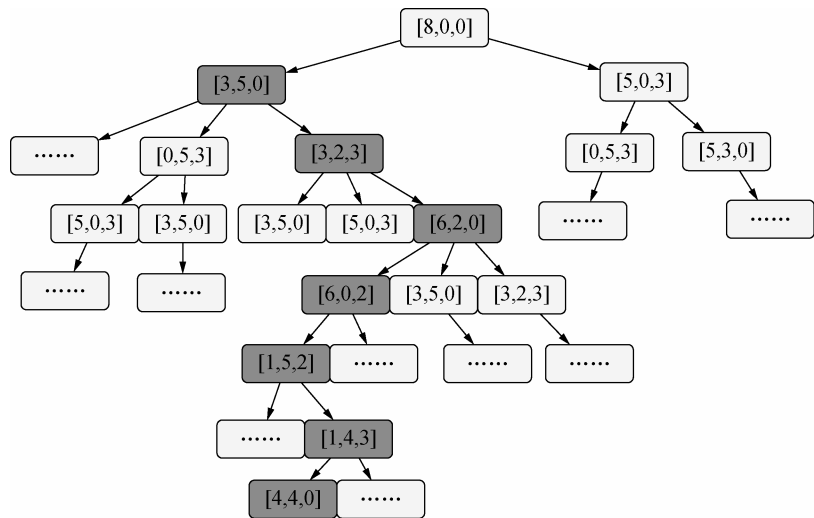
图 5-1 状态树结构示意图
