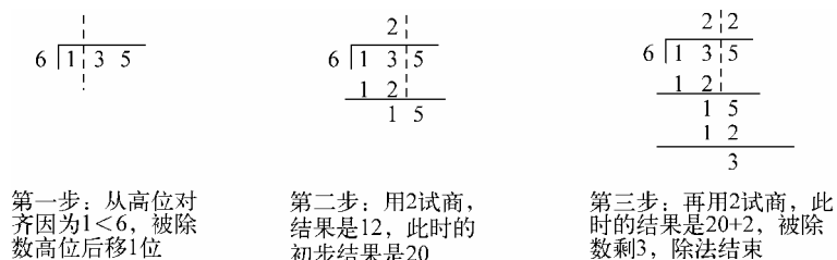
图 17-3 十进制除法计算过程
