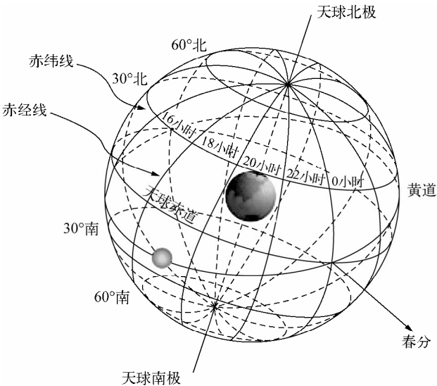
图 11-1 天球概念示意图
