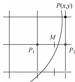
图 14-15 中点法对下部区域处理示意图
