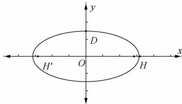
图 14-12 椭圆的对称性
