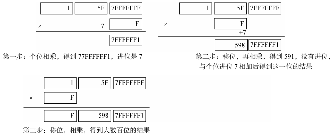
图 17-2 大数乘法计算过程
