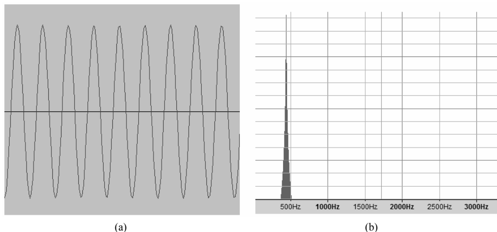
图 15-1 440Hz 正弦波在时域和频域内的形态
