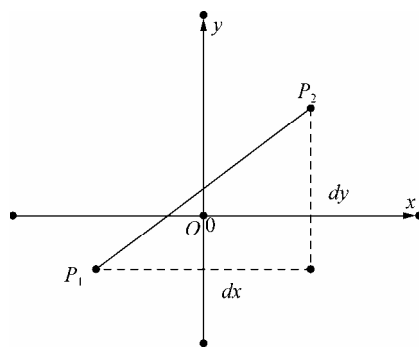
图 14-1 平面两点距离计算示意图
