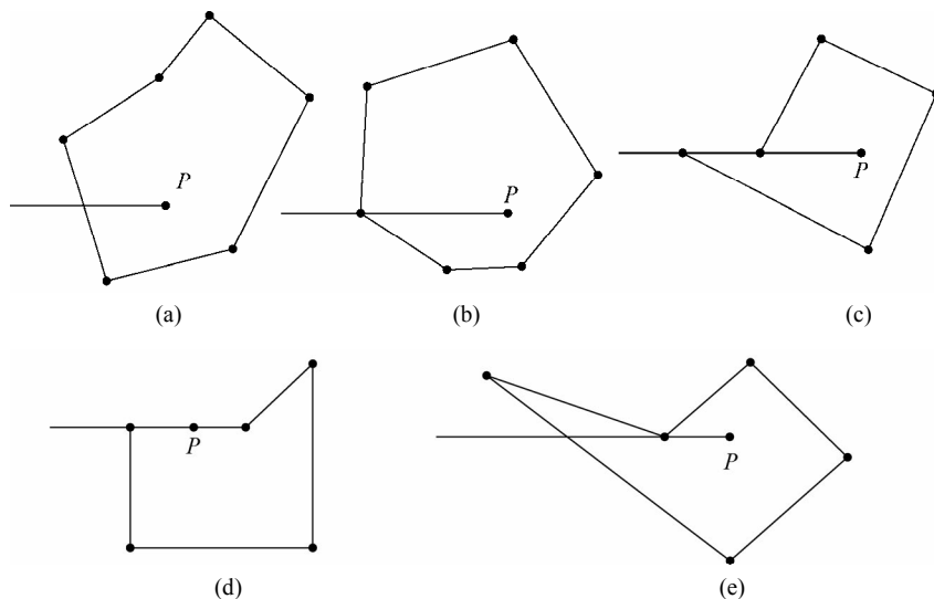
图 14-4 射线法可能遇到的各种交点情况
