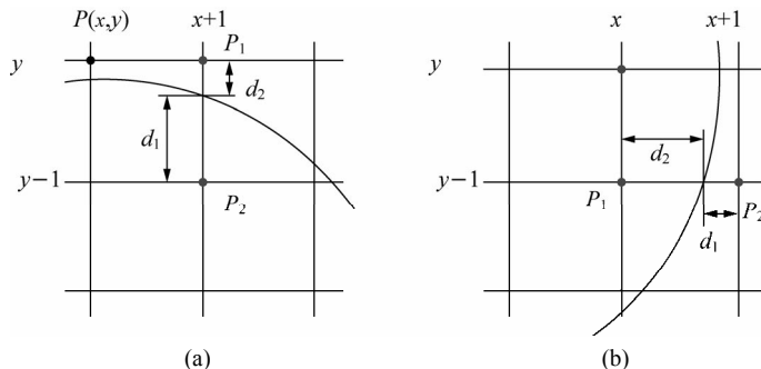
图 14-16 Bresenham 椭圆生成算法判别式
