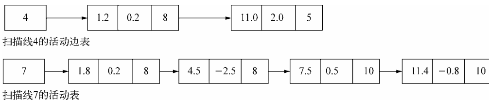
图 14-21 扫描线的活动边表示意图
