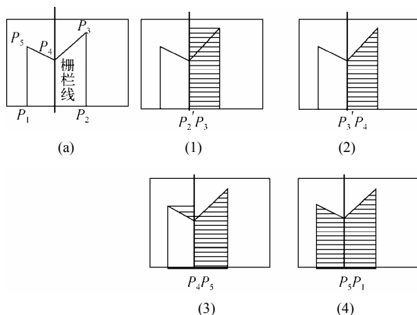
图 14-26 栅栏填充算法的处理过程
