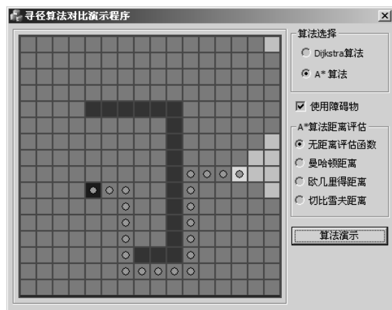
图 21-4 A*算法退化为 Dijkstra 算法的效果
