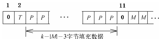
图 18-1 PKCS #1 1.5 填充模式
