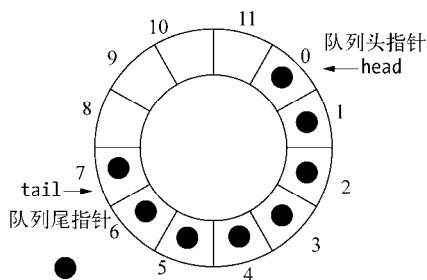
图 1-1 环形队列示意图
