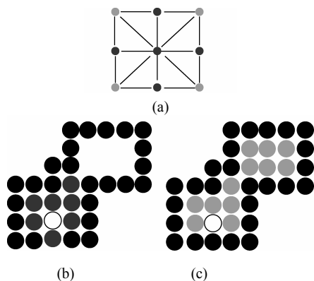
图14-17 “4-联通”和“8-联通”填充效果图
