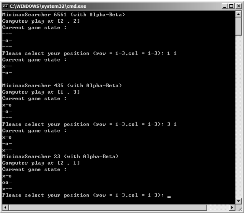
图 23-5 简单的井字棋游戏
