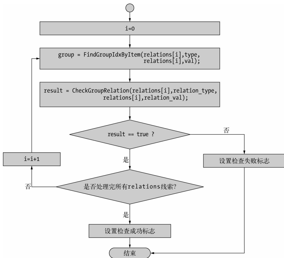
图 8-2 “组”相邻关系线索检查流程图
