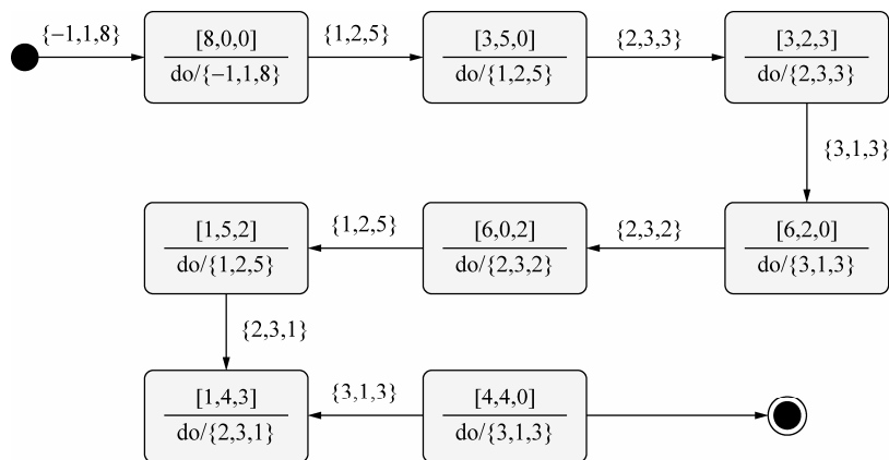
图 5-2 组合状态转换过程示意图
