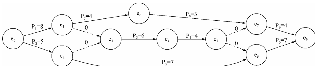
图 9-3 由事件顶点和活动边组成的 AOE 网
