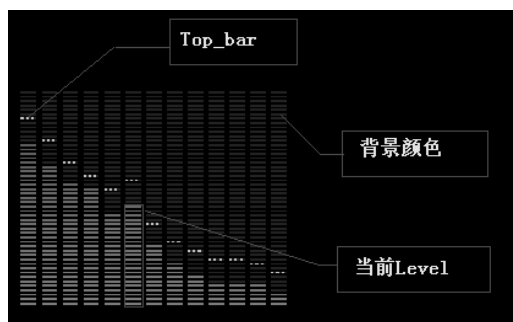
图 15-6 频谱显示的主要元素
