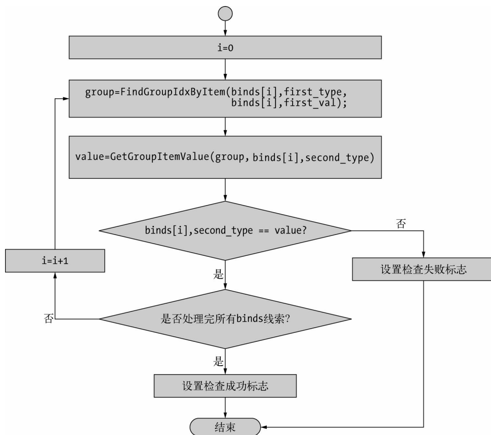
图 8-1 绑定关系线索检查的流程图
