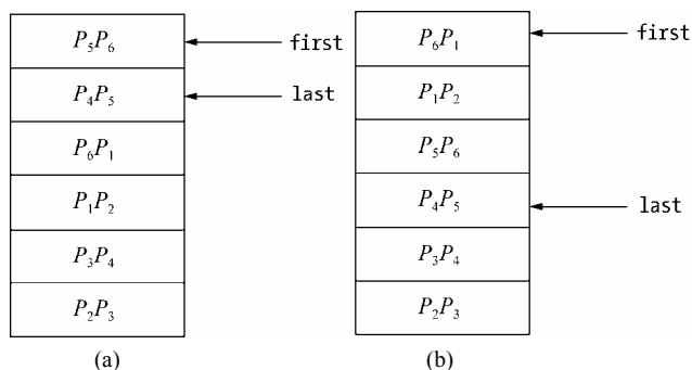
图 14-24 改进的活动边表结构
