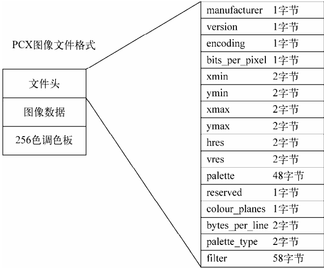
图 10-1 PCX 文件结构示意图
