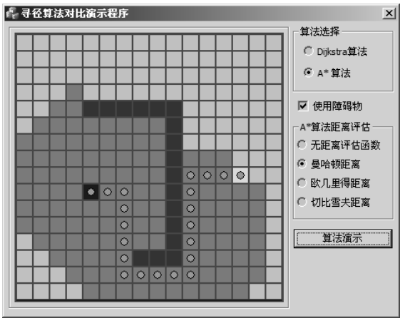
图 21-6 使用曼哈顿距离的 A*算法效果
