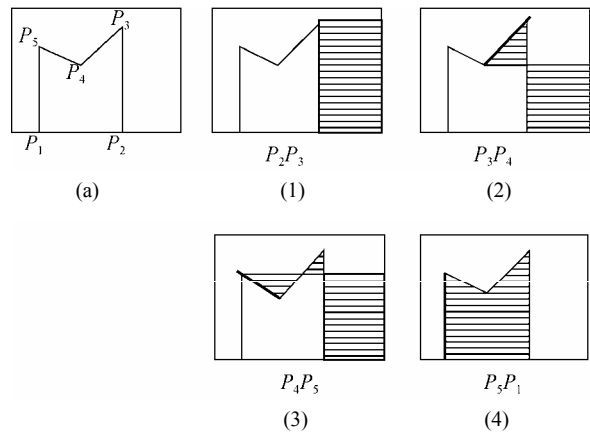
图 14-25 边缘填充算法的处理过程
