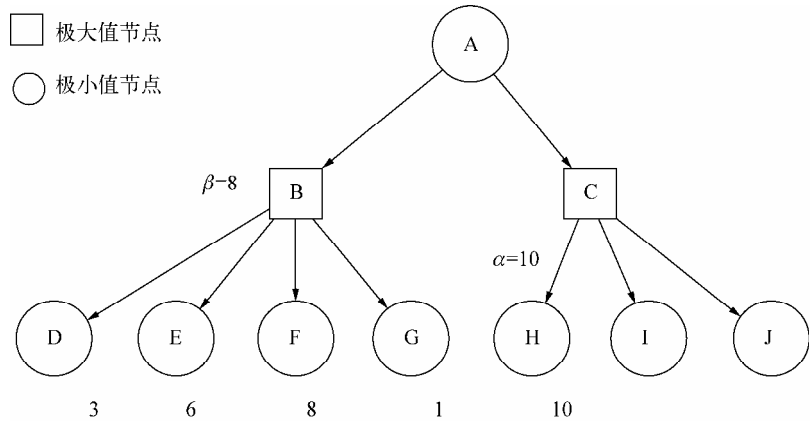
图 23-3 “ \beta 剪枝” 过程示意图
