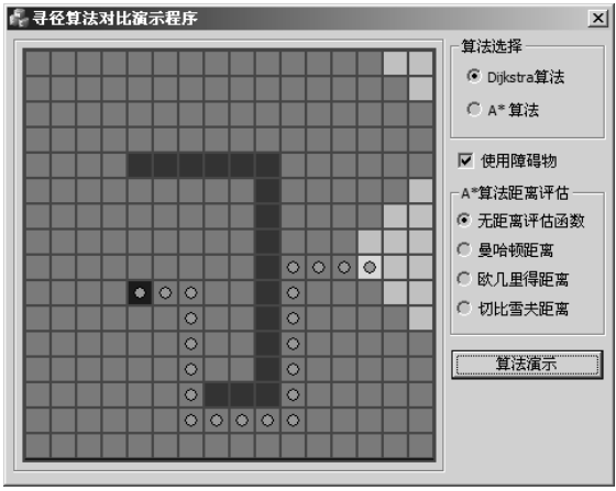
图 21-2 Dijkstra 算法搜索效率图示（有障碍物的情况）
