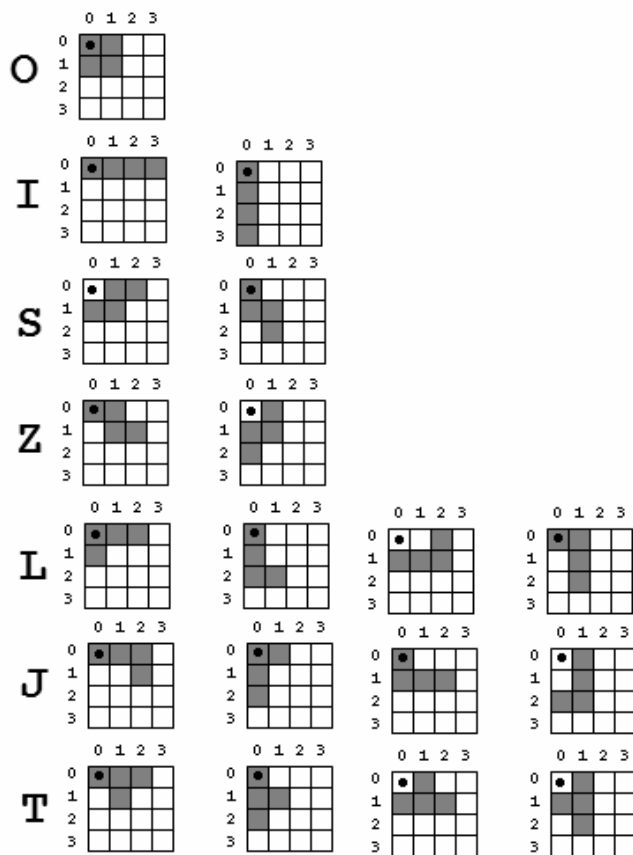
图 22-7 板块形状数据定义示意图
