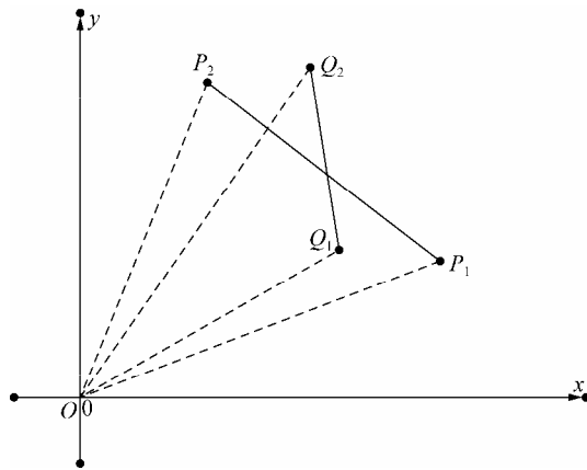
图 14-3 直线段跨立试验示意图
