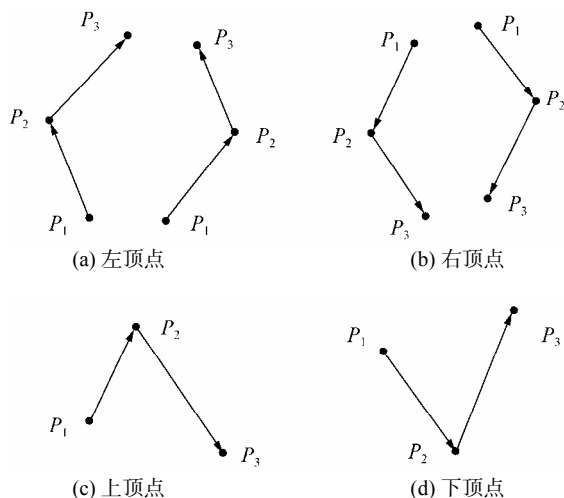
图 14-23 多边形顶点的四种类型
