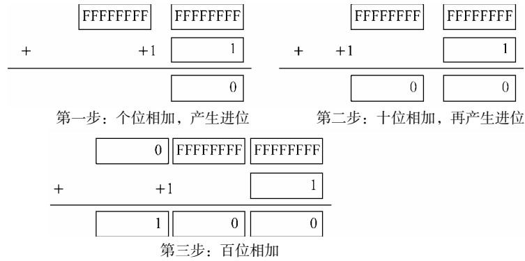
图 17-1 大数加法计算过程
