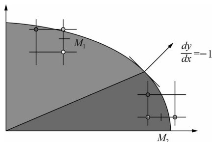
图 14-13 第一象限椭圆弧示意图
