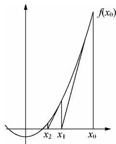
图 13-1 牛顿迭代法逼近示意图
