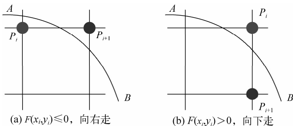
图 14-11 正负法判定示意图
