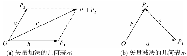
图 14-2 矢量加法和矢量减法的几何意义
