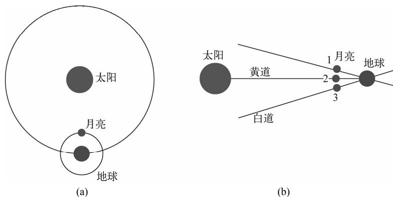
图 11-3 日月天文现象示意图
