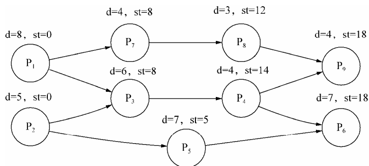
图 9-2 由活动顶点组成的 AOV 网
