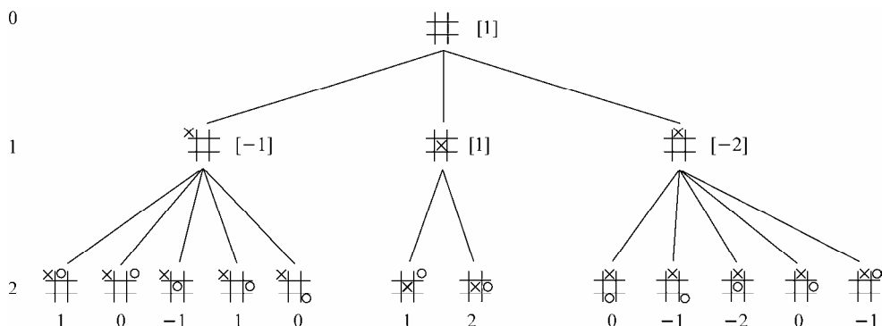
图 23-1 井字棋游戏极大极小博弈树示意图
