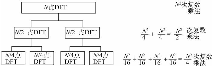
图 15-2 基 2 FFT 分解与计算量
