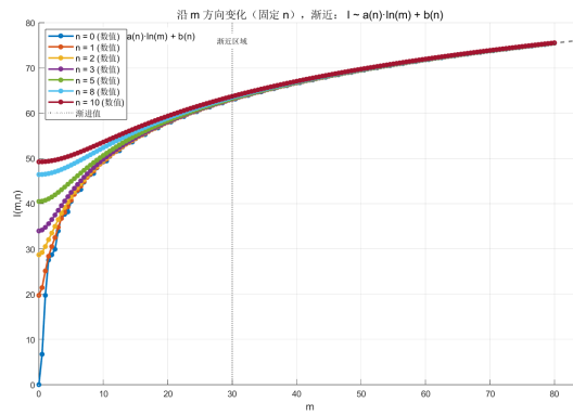
图 1 纯电阻网格积分值 I(m, n) 固定 n 随 m 的变化
