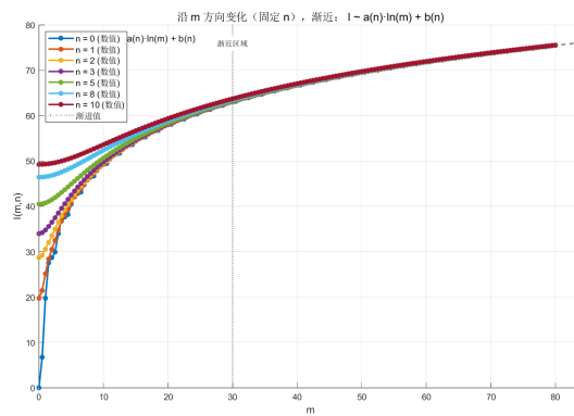
图 1 纯电阻网络积分值 I(m, n) 固定 n 随 m 的变化
