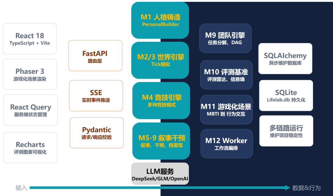
Figure 1: Life Lab 系统技术架构图：表现层（React + Phaser 3）→ 接口层（FastAPI + SSE）→ 引擎层（8 大引擎）→ 数据层（SQLAlchemy + SQLite）。LLM 服务通过 OpenAI 兼容 API 接入。
