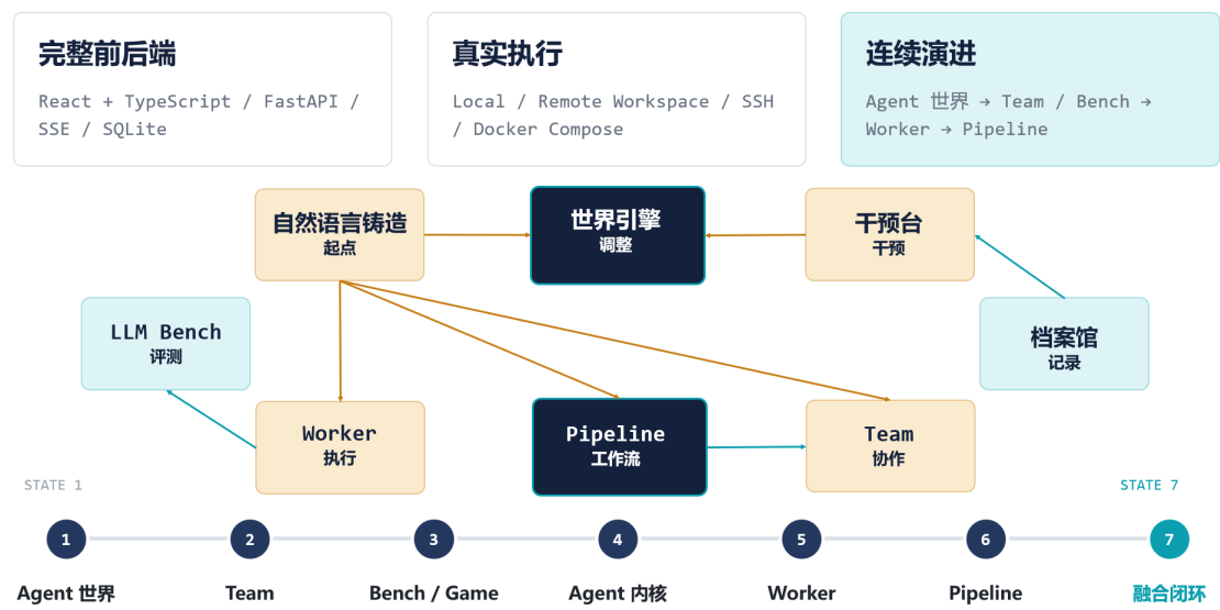
Figure 2: Life Lab 七阶段连续演进：从 Agent 世界（STATE 1）到融合闭环（STATE 7），涵盖完整前后端、真实执行、LLM Bench、Pipeline 工作流等核心能力。
