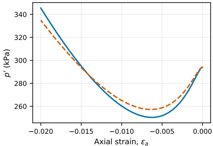
(d) Pore-pressure accumulation
