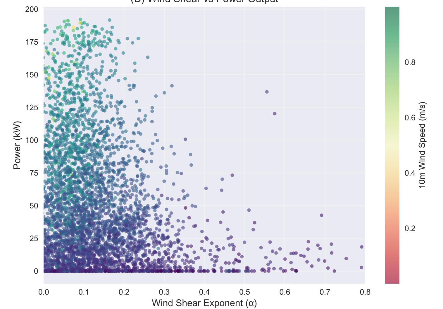
(D) Wind Shear vs Power Output
