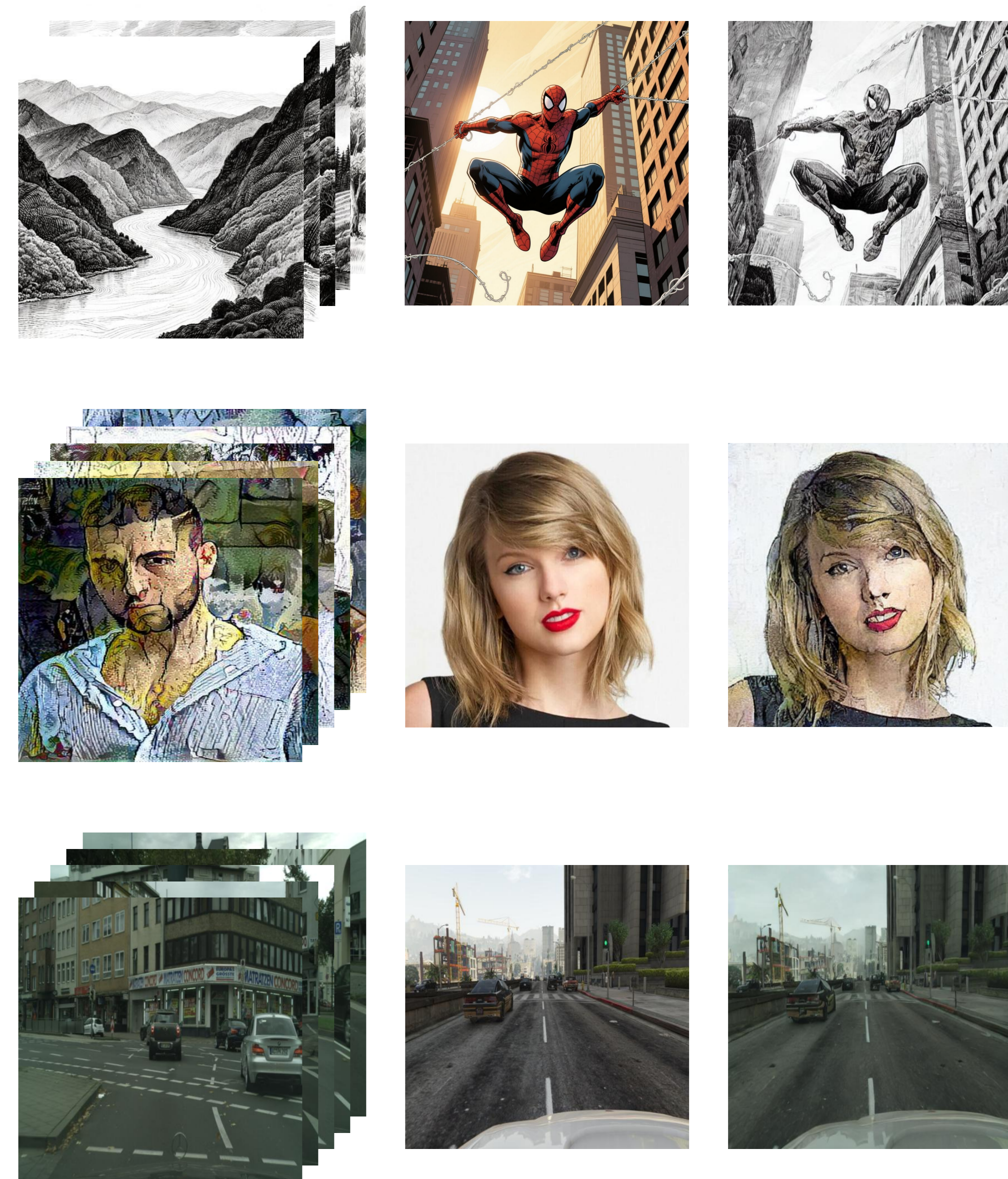
V-Shuffle (Ours)
