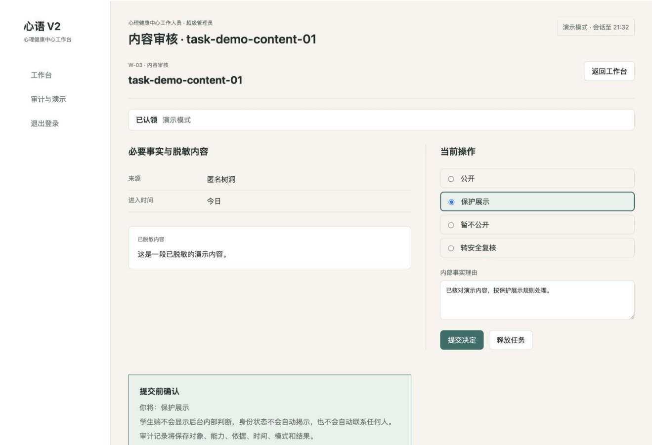
图 40：审核提交确认功能界面
