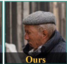
Ours
