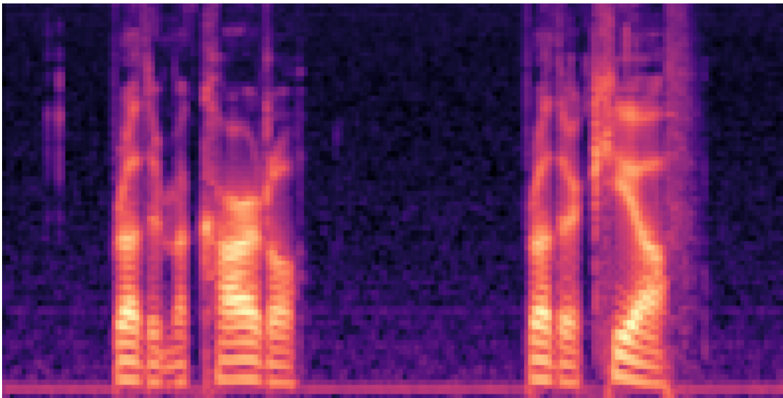
Opus + LBRR (8.0 kbps)
