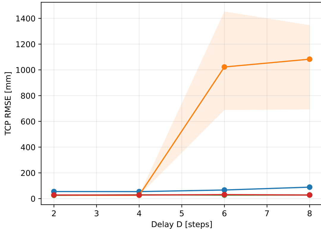
circle
