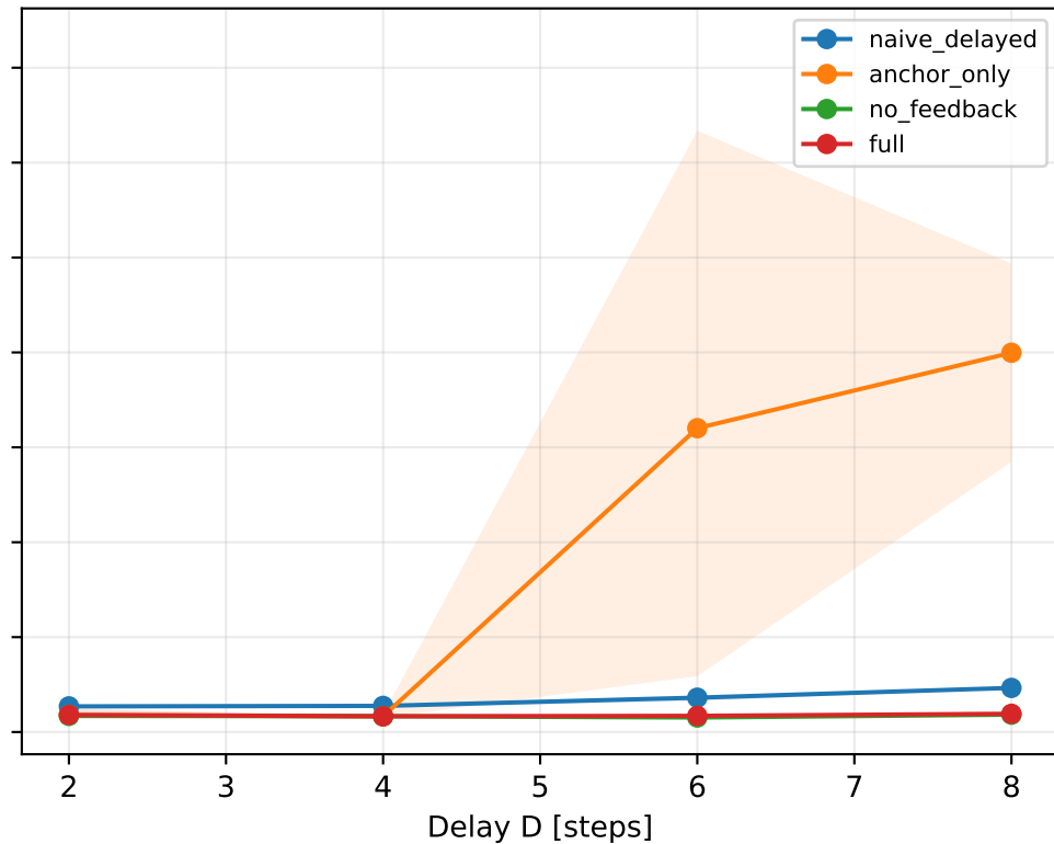
fast_ellipse
