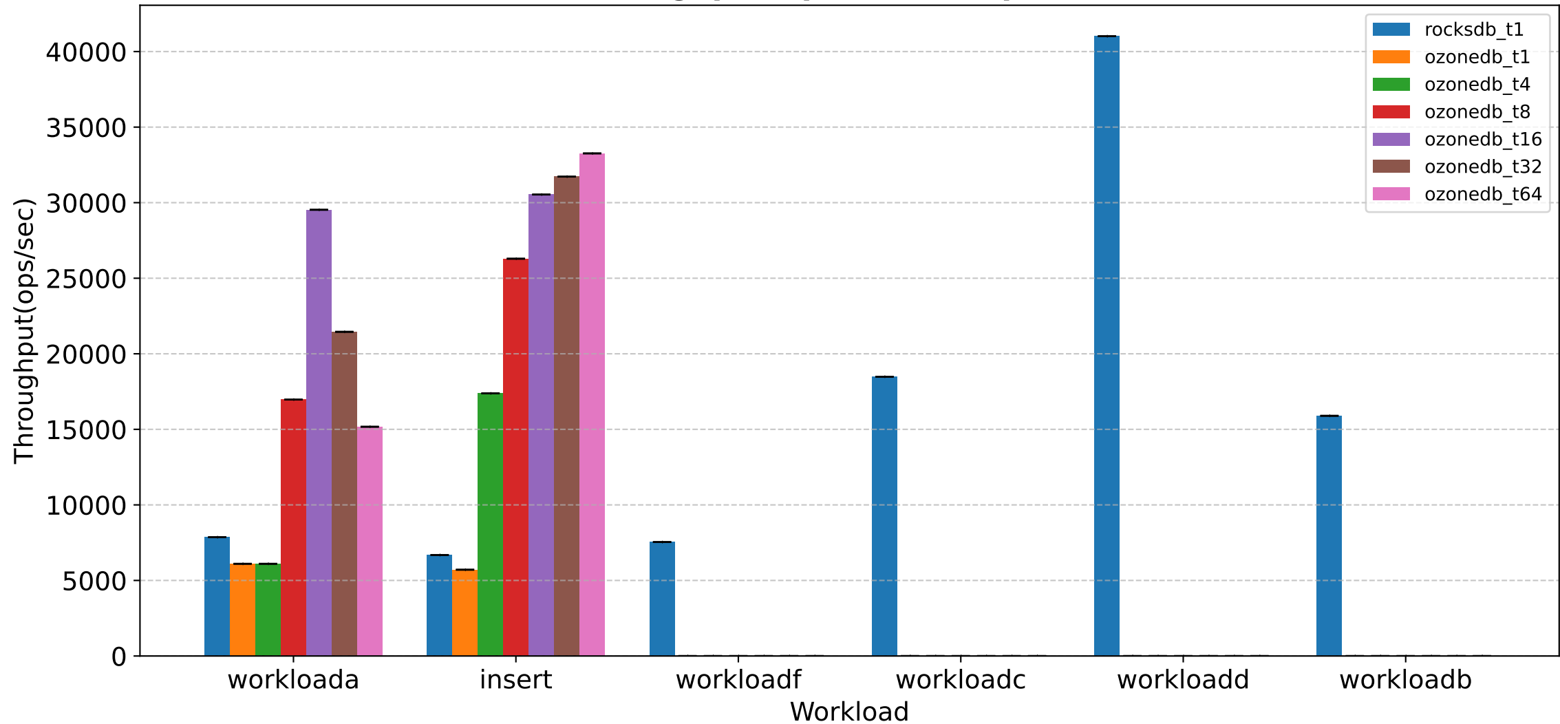
Throughput(ops/sec) Comparison
