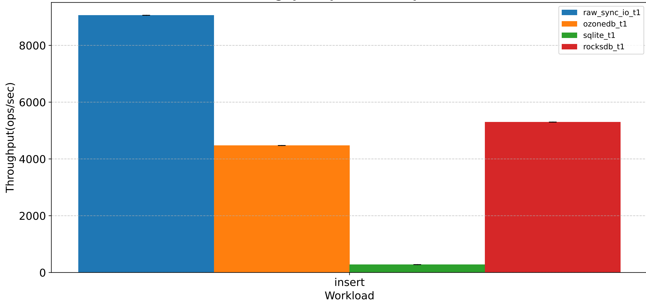
Throughput(ops/sec) Comparison
