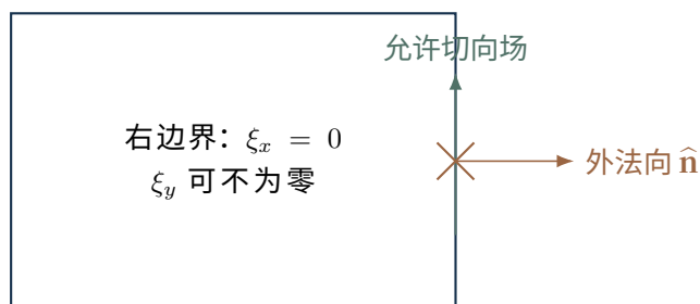
图 2 零法向条件不要求整条边界的所有电场分量都为零。
