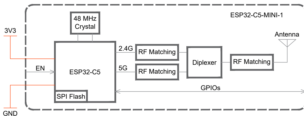
图 1: ESP32-C5-MINI-1 功能框图
