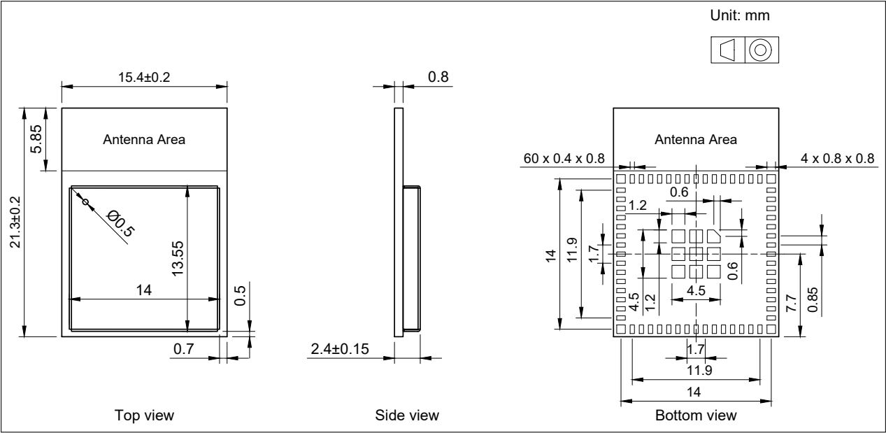
图 6: ESP32-C5-MINI-1 模组尺寸
