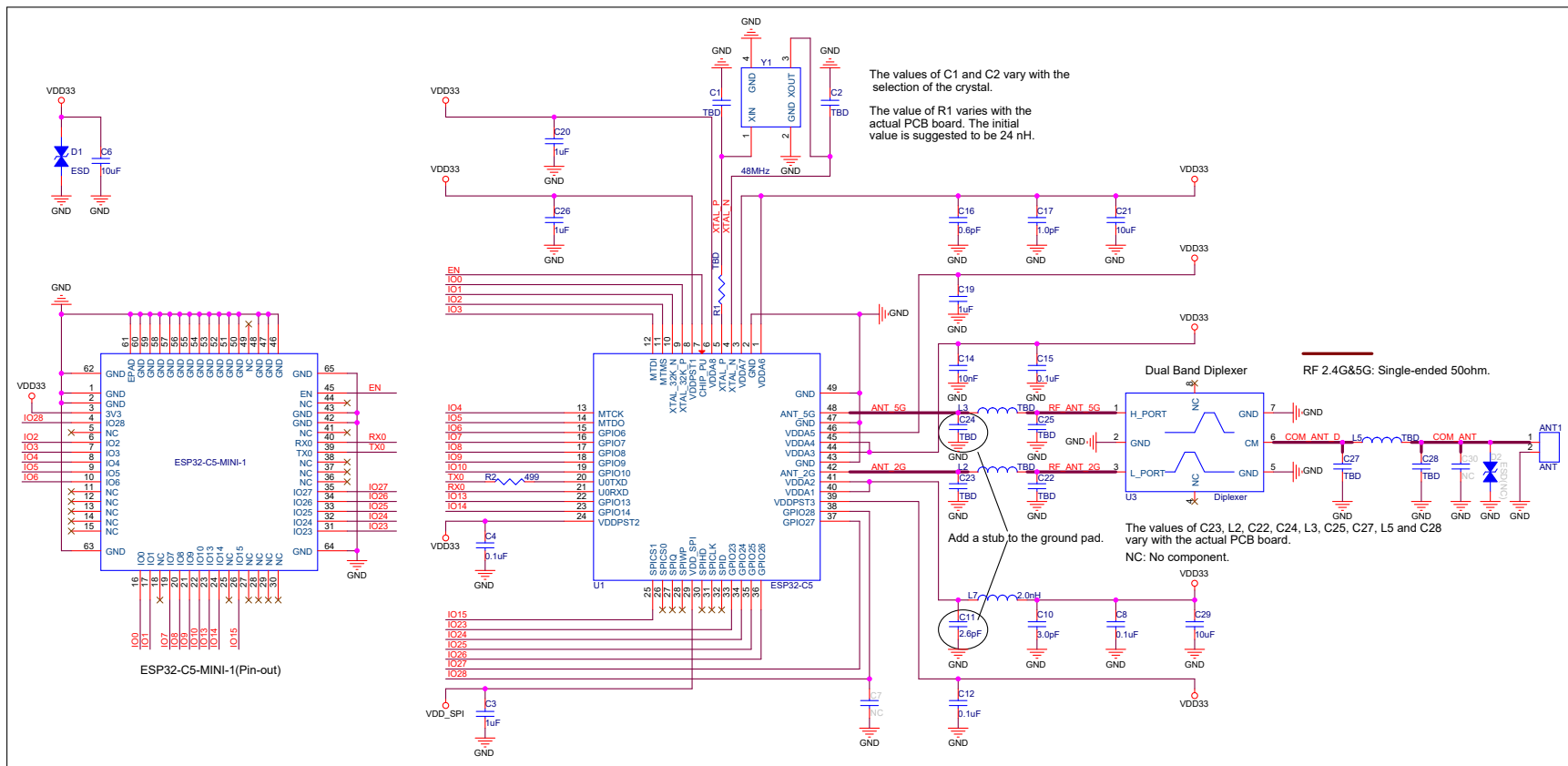
图 4: ESP32-C5-MINI-1 原理图
