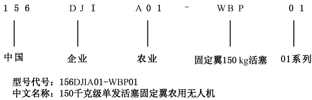
图 2 民用无人机系统型号命名示例
