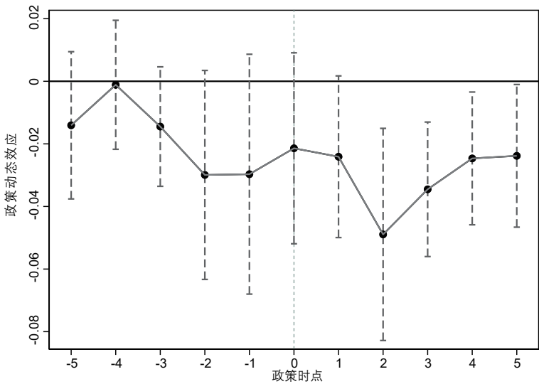
图 3 事前平行趋势评估
