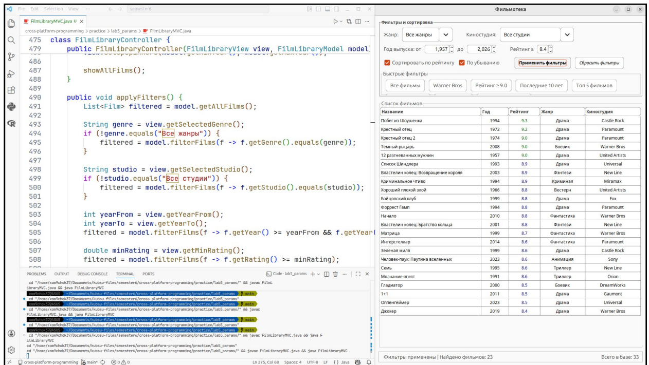
Рисунок 5 — Комбинирование предикатов
