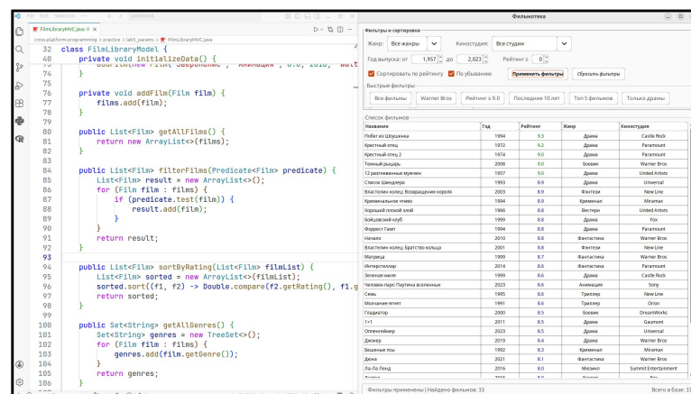
Рисунок 2 — Применение интерфейса-предиката
