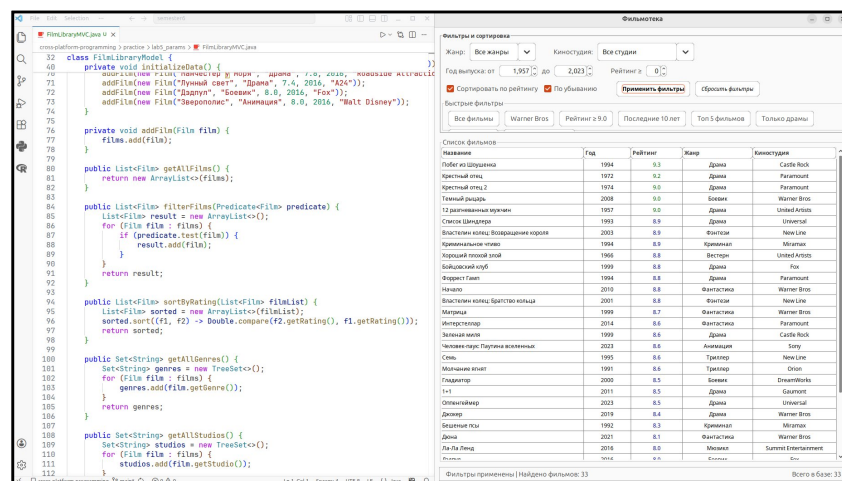
Рисунок 1 — Паттерн «Стратегия»
